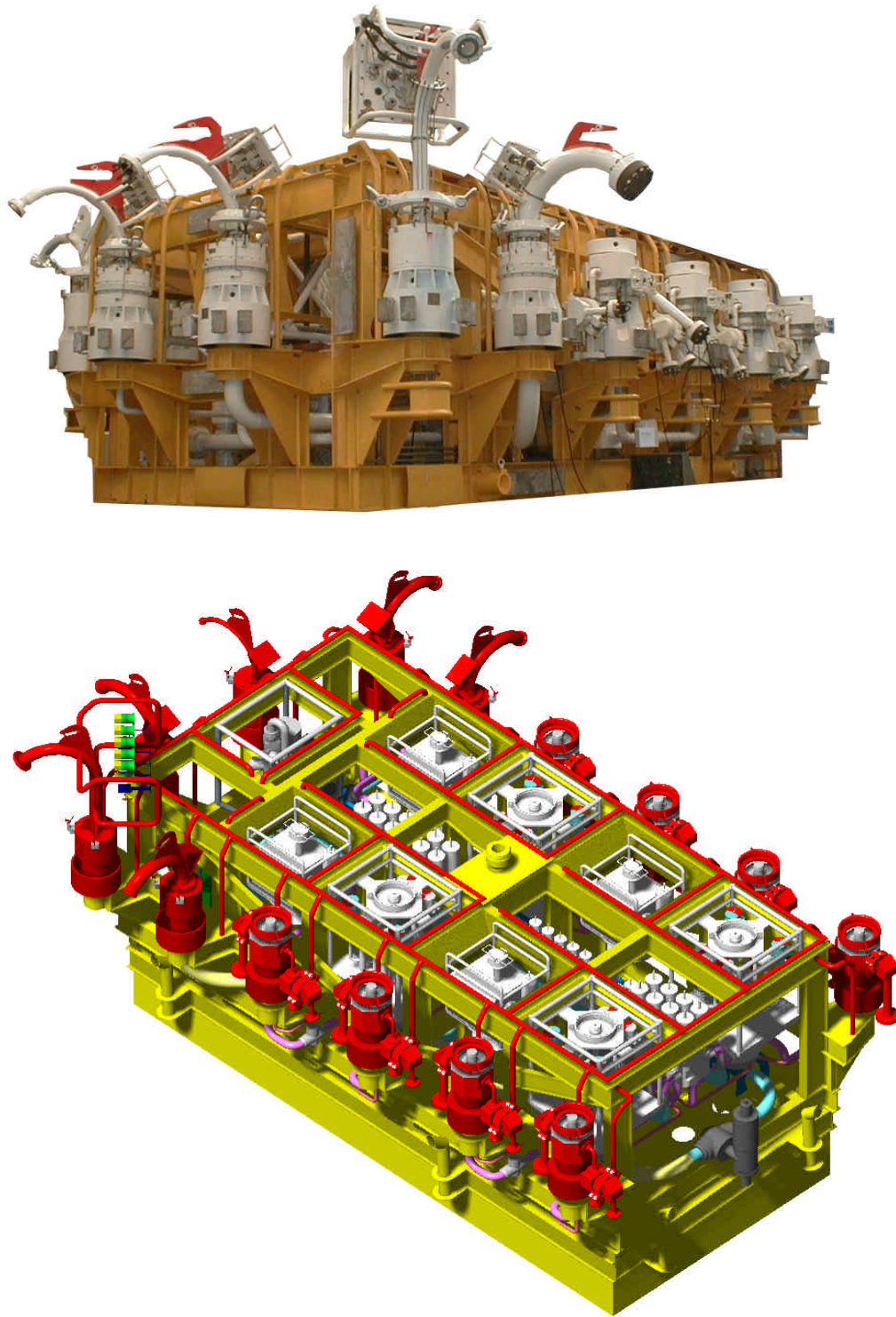
Figura A.9 – Manifold Submarino do Campo de Marimba
