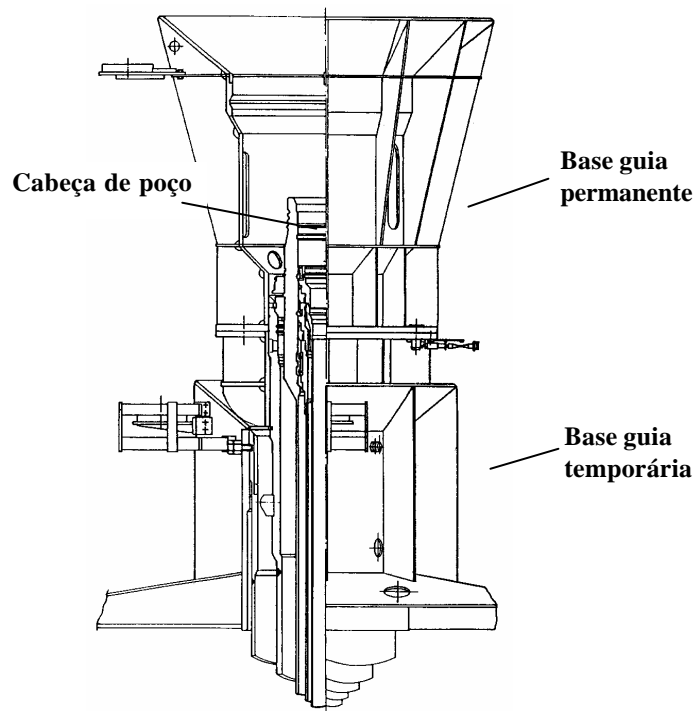
Figura A.1 - Base guia e Cabeça de Poço
