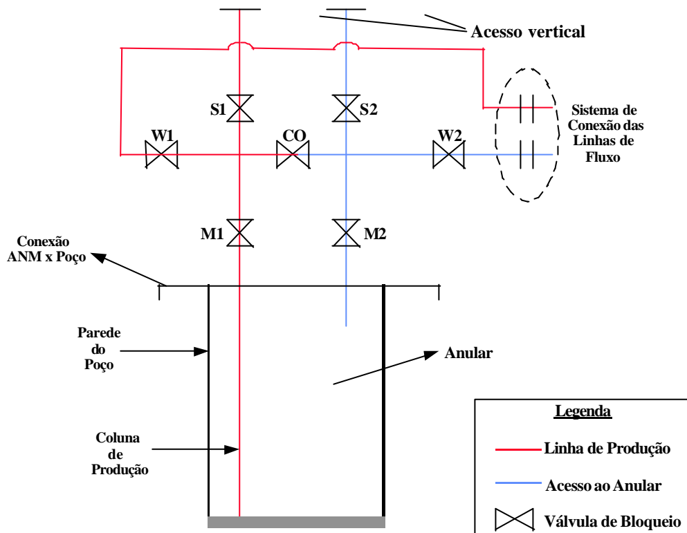
Figura A.2 - Diagrama genérico de uma árvore de natal
