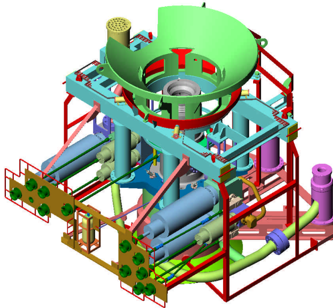
Figura A.4 - Árvore de Natal Molhada de Produção - Horizontal LDA 3000m (ANM-H)
