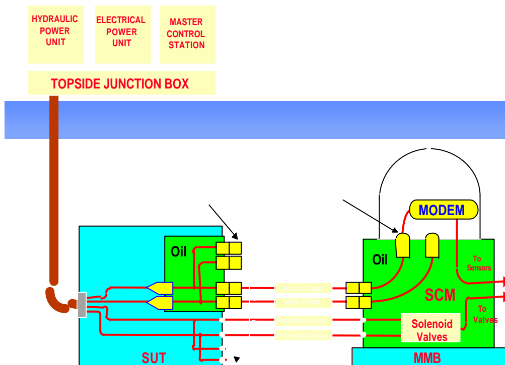
Figura A.8 – Esquema Típico de Sistema de Controle Submarino em Manifolds
