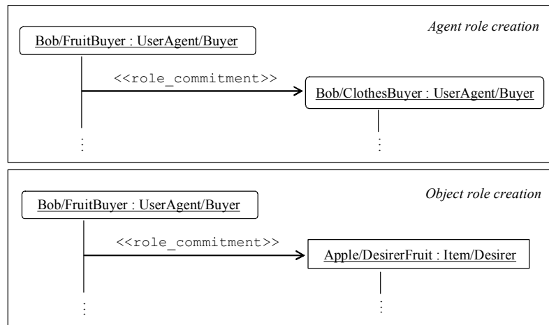
Figura 27 – Comprometendo-se com um papel.
