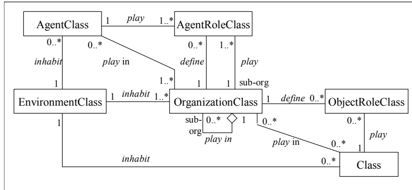
Figura 23 - As associações entre as metaclasses que representam as entidades do TAO.
