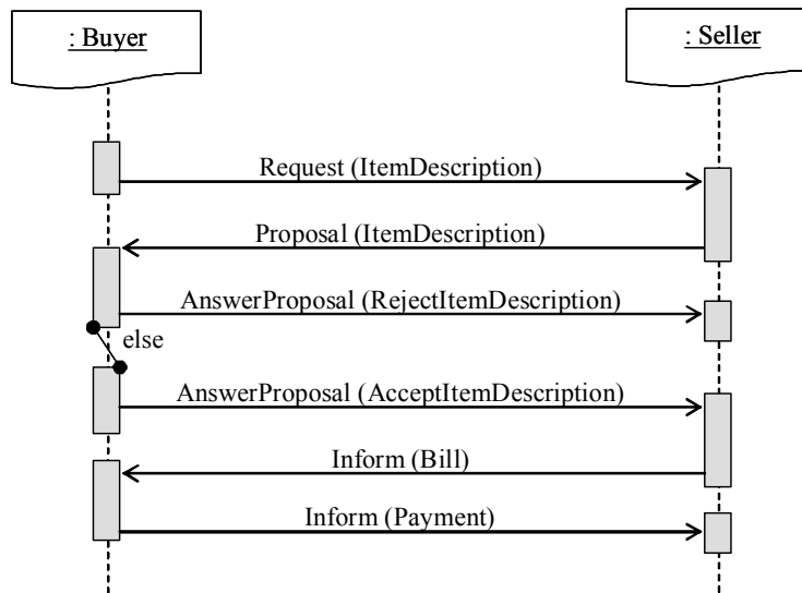
Figura 32 – O protocolo de negociação.
