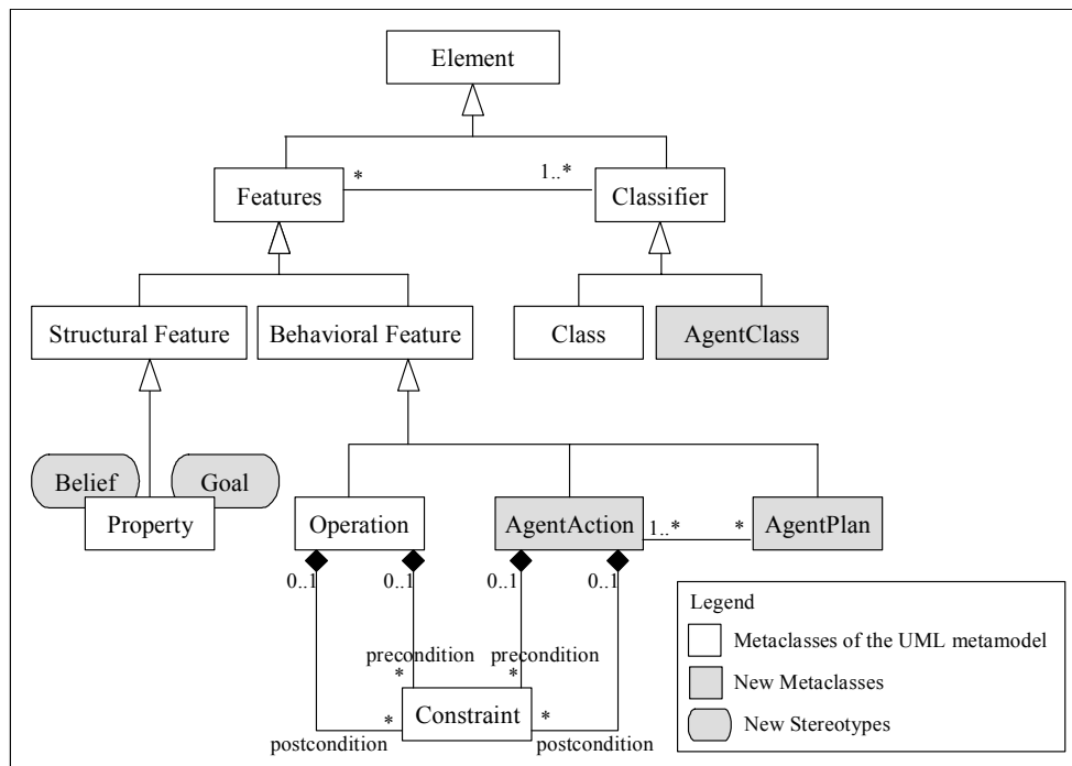
Figura 12 – O metamodelo de UML estendido para incorporar agentes e suas propriedades.
