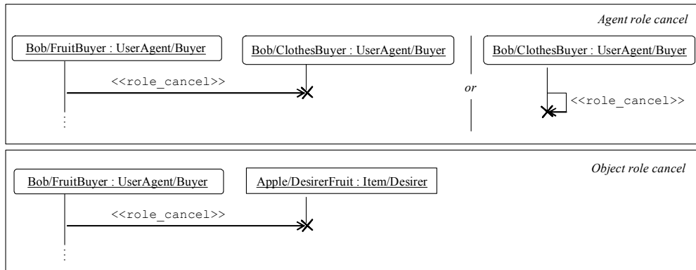
Figura 28 – Cancelando um papel.
