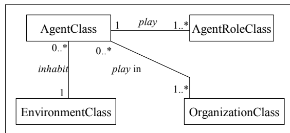
Figura 13 – As associações entre AgentClass e outras metaclasses.
