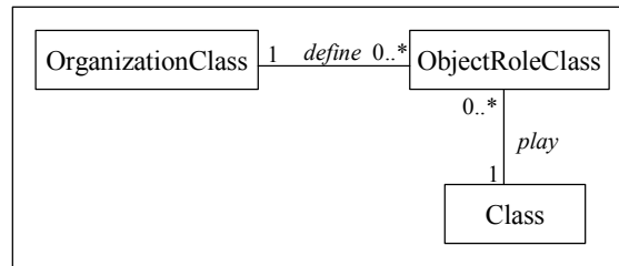
Figura 15 – As associações entre ObjectRoleClass e outras metaclasses.
