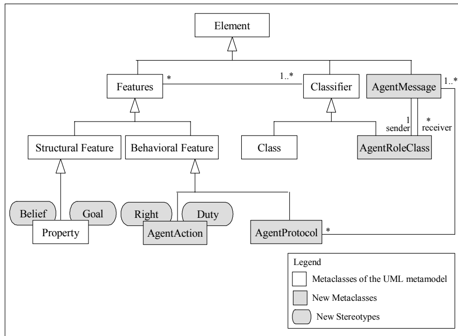
Figura 16 – O metamodelo de UML estendido para incorporar papéis do agente e suas propriedades.
