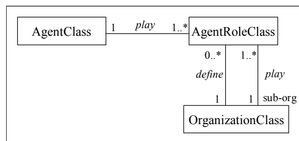
Figura 17 – As associações entre AgentRoleClass e outras metaclasses.
