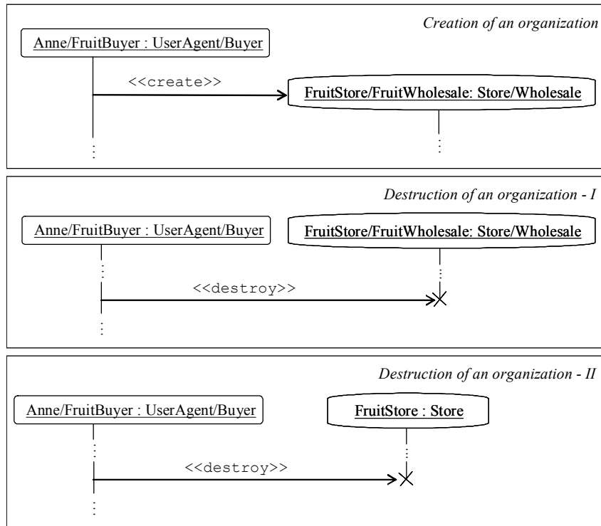
Figura 26 – Criação e destruição de uma organização.
