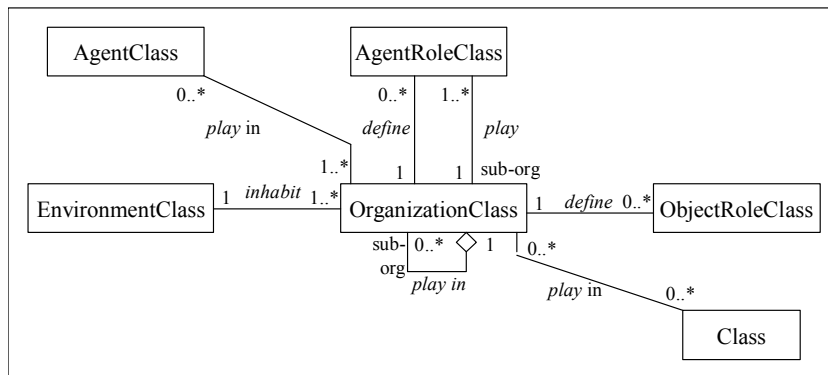
Figura 19 – As associações entre OrganizationClass e outras metaclasses.
