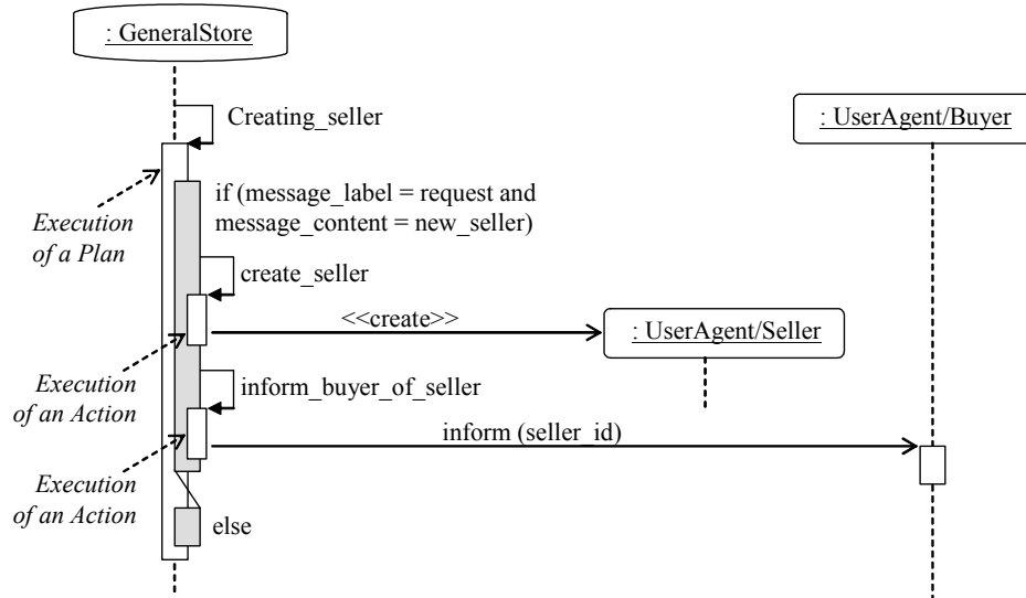
Figura 31 – Modelando a execução de um plano e suas ações.
