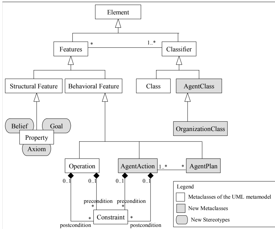
Figura 18 – O metamodelo de UML estendido para incorporar organização e suas propriedades.
