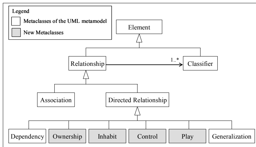
Figura 24 – O metamodelo de UML estendido para incorporar os relacionamentos MAS-ML.
