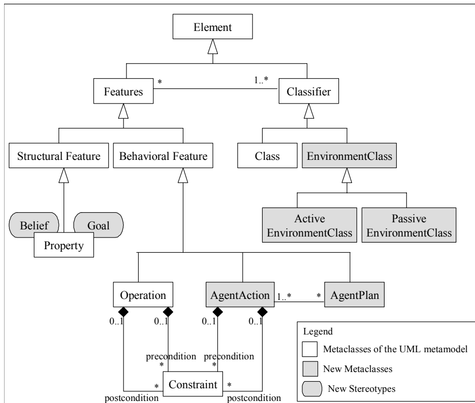
Figura 20 – O metamodelo de UML estendido para incorporar ambientes e suas propriedades.
