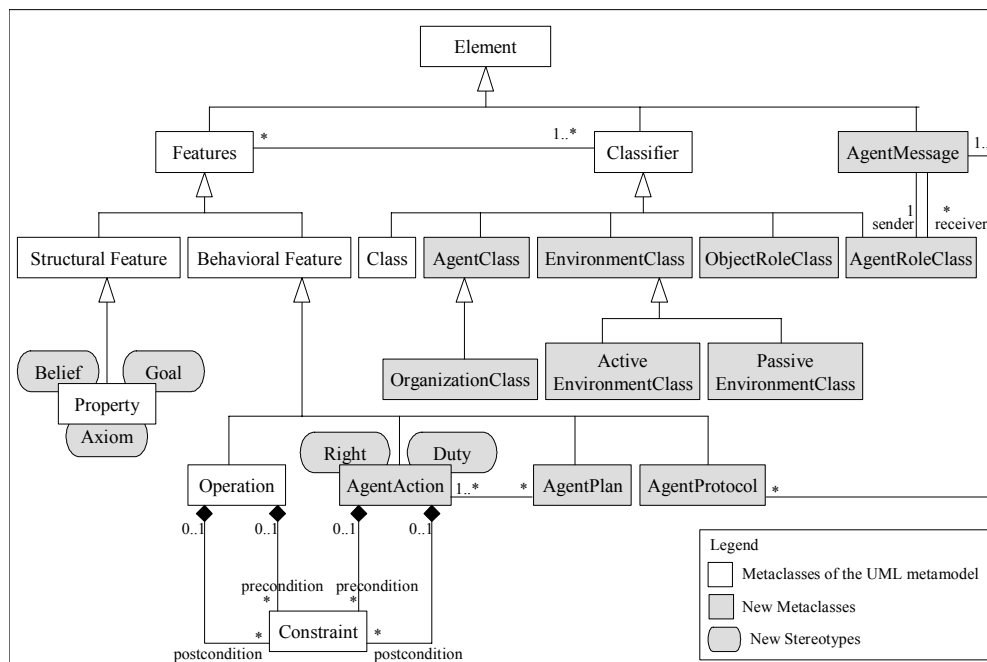
Figura 22 – O metamodelo de UML estendido para incorporar as entidades da MAS-ML e suas propriedades.
