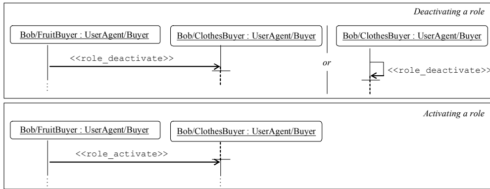
Figura 29 – Ativando e desativando um papel.
