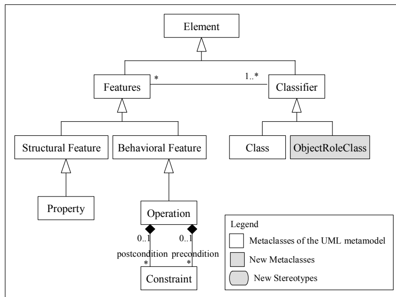
Figura 14 – O metamodelo de UML estendido para incorporar papéis de objeto.
