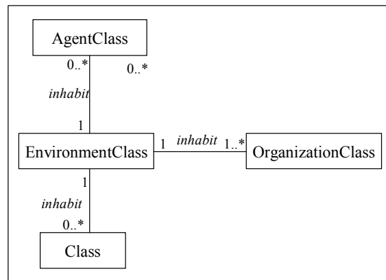
Figura 21 – As associações entre EnvironmentClass e outras metaclasses.
