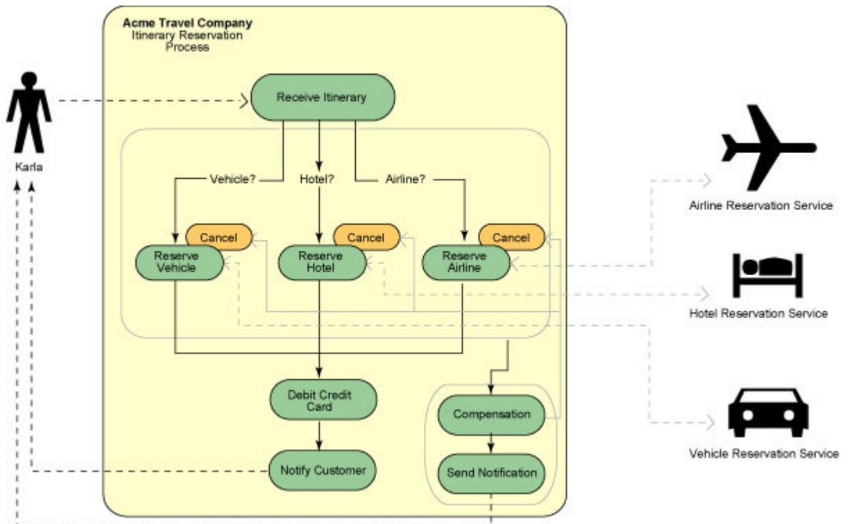
Figura 4 - Exemplo de composição de serviços
