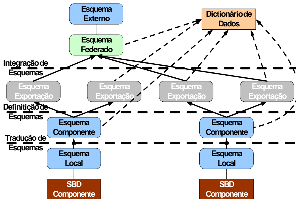
Figura 17. Processo de desenvolvimento de baixo para cima de um SBD Federado [SL90].
