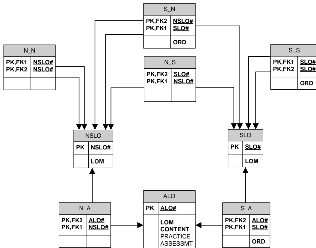
Figura 16. Modelo Relacional de Objetos de Aprendizado [PPM03]
