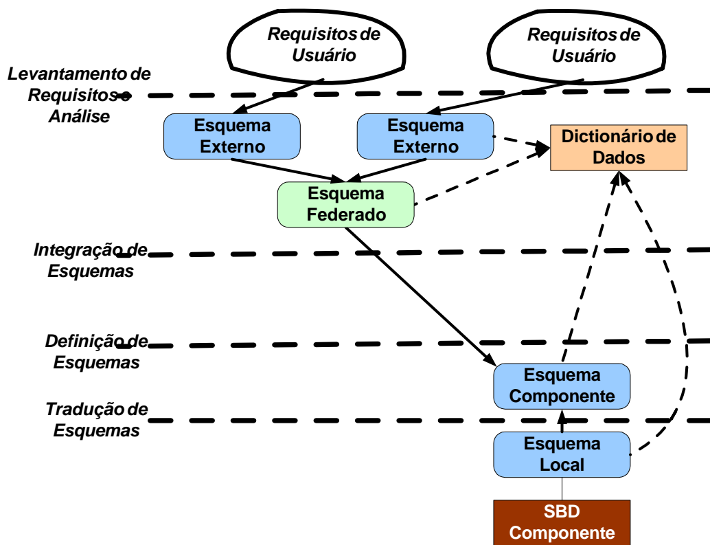
Figura 18. Processo de desenvolvimento de um SBDF de cima para baixo [SL90].
