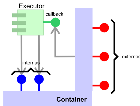
Figura 2.3: Interfaces do contêiner CCM.
