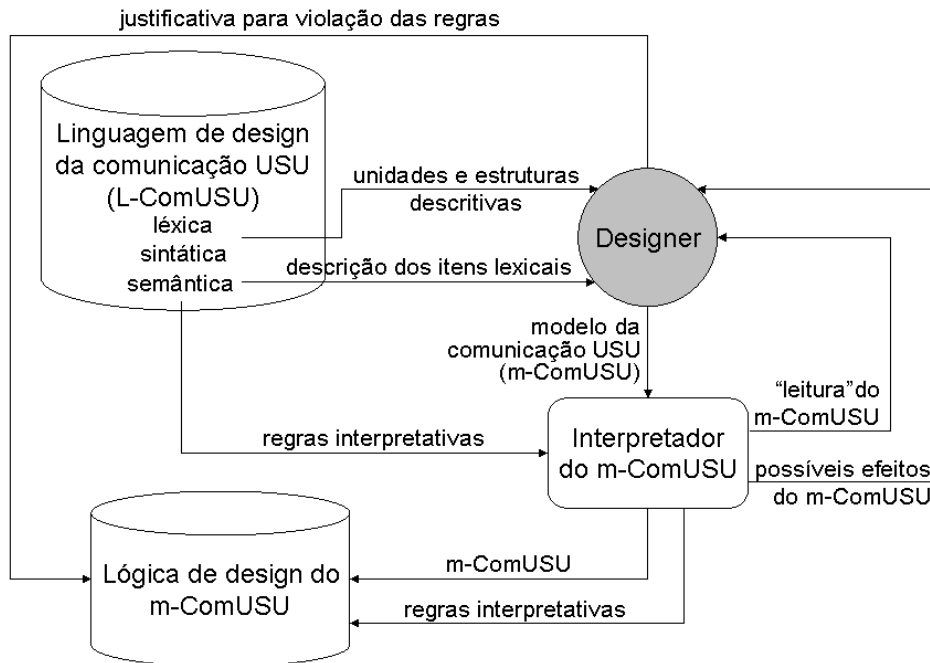
Figura 11 - Modelo de arquitetura da Manas
