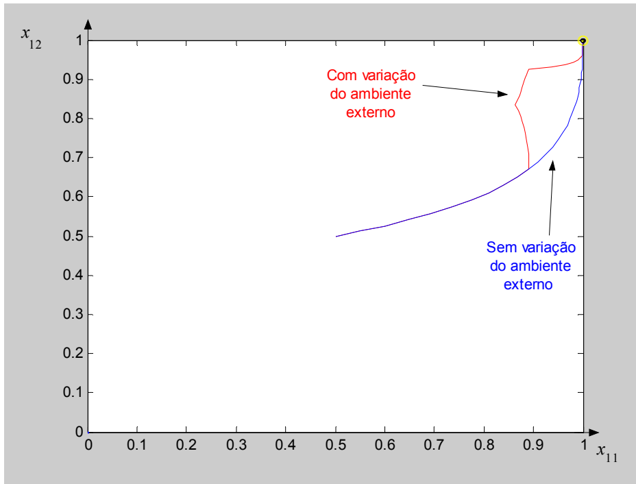
Figura 5-9 – Interferência do ambiente externo na matriz de payoff
