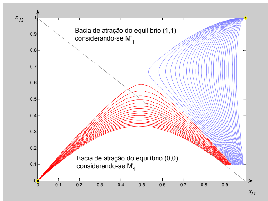
Figura 5-14 – Distorção na bacia de atração provocada por mudanças no ambiente
