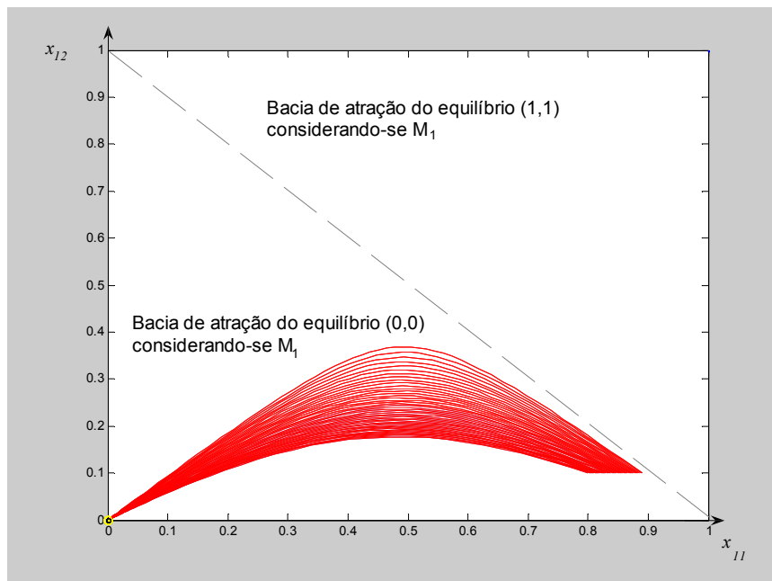
Figura 5-13 – Bacias de atração originais
