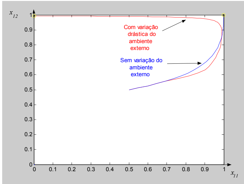
Figura 5-10 – Mudança de órbita por influência externa
