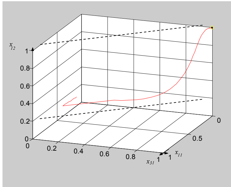
Figura 5-8 – Estratégia mutante melhor que estratégia original
