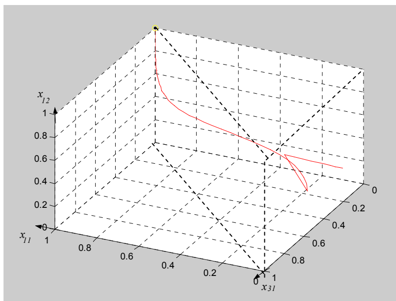
Figura 5-7 – Órbita com mutante pior que a residente.
