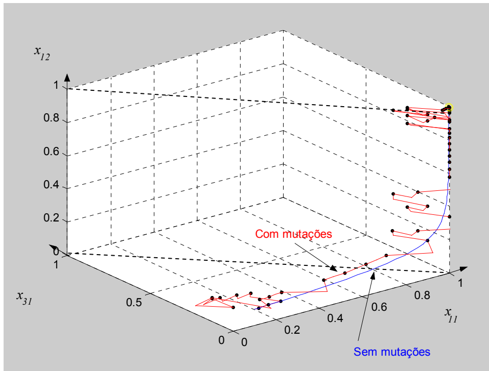
Figura 5-3 – Órbitas com mutações na mesma bacia de atração
