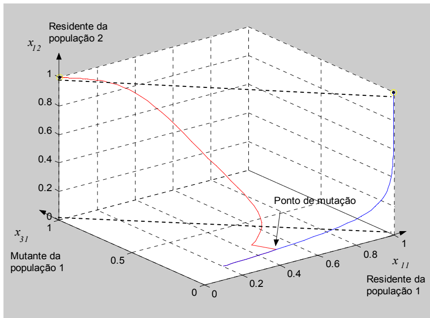
Figura 5-1 – Órbita sem e com mutação
