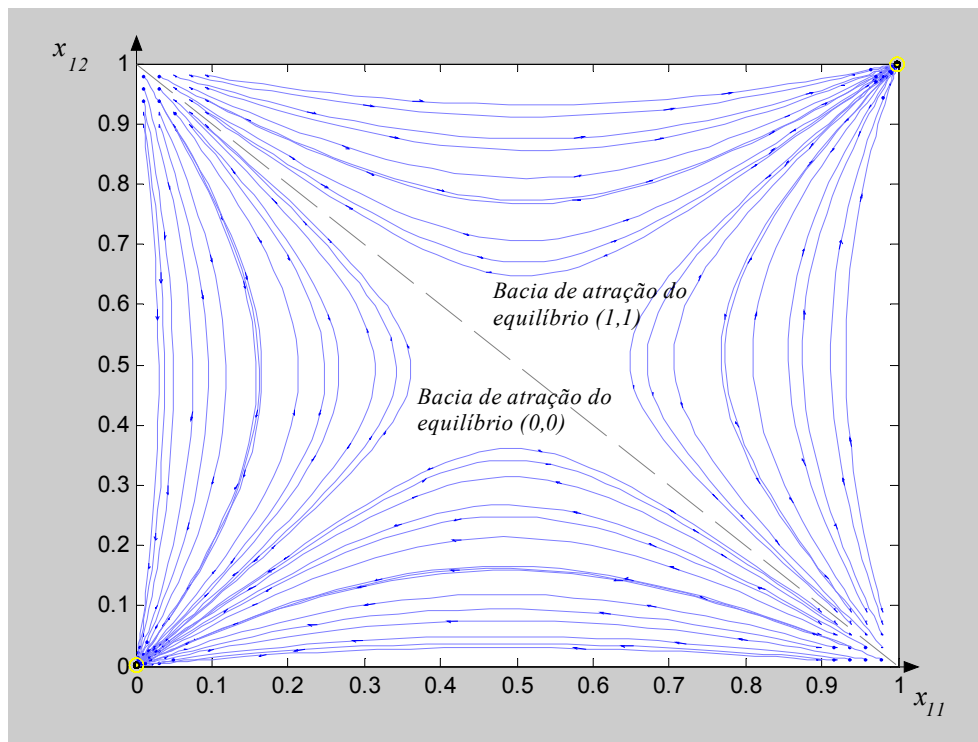
Figura 5-4 – Duas bacias de atração para os equilíbrio (e_1^1, e_2^1) e (e_1^2, e_2^2)
