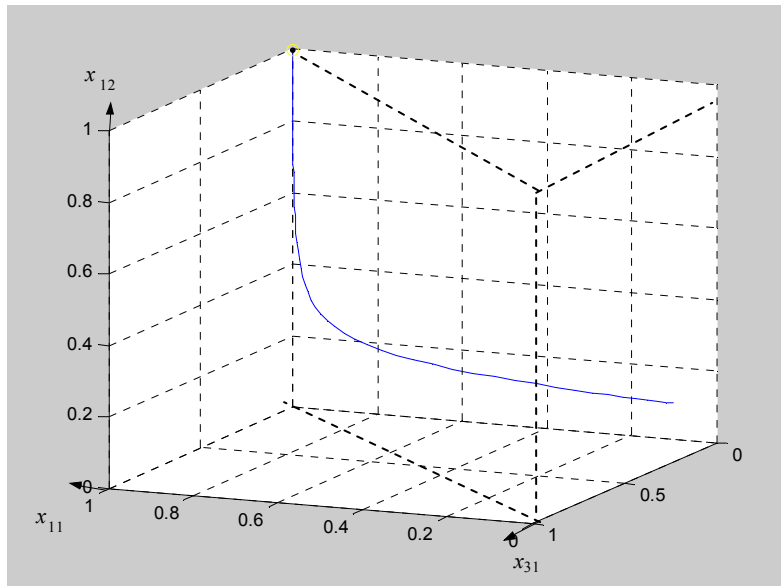
Figura 5-6 – Órbita na face original x_{11} e x_{12}
