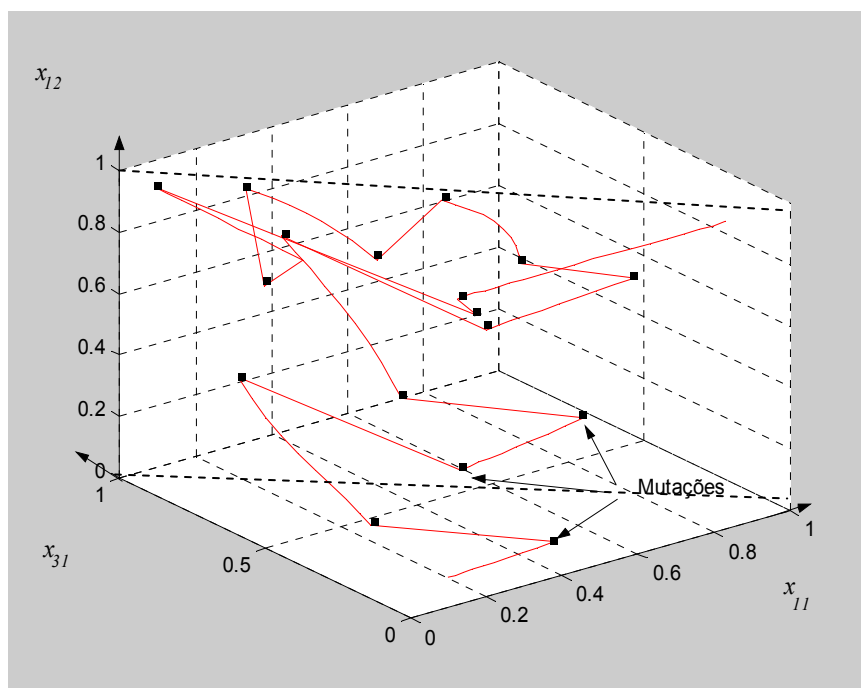
Figura 5-2 – Órbita com mutações frequentes
