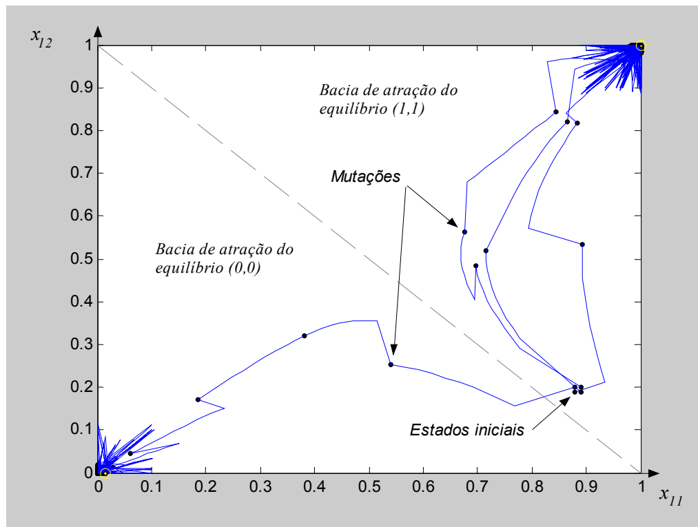
Figura 5-5 – Órbitas que mudam de bacia de atração por efeito de mutações
