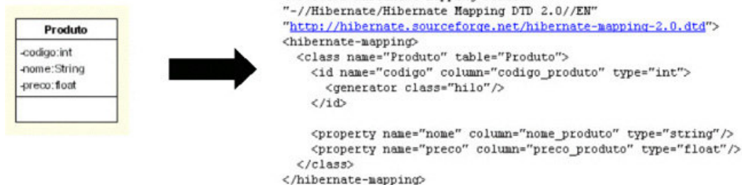
Figura 39 - Arquivo XML contendo o mapeamento tabela-classe do Framework Hibernate
