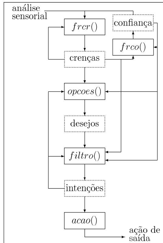
Figura 4.1: Diagrama esquemático de uma arquitetura de crenças, desejos e intenções com confiança genérica
