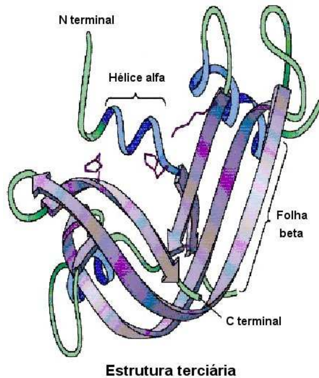
Figura 3.4 Exemplo de estrutura terciária de uma proteína.
