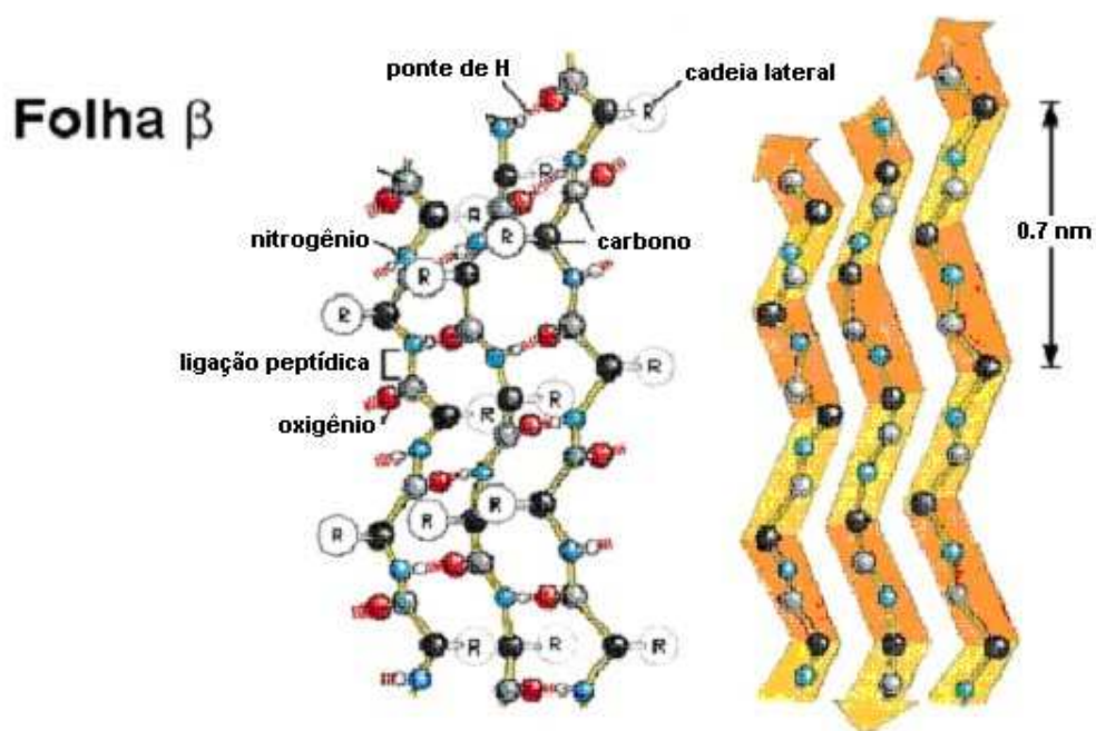
Figura 3.3 Exemplo de uma estrutura do tipo folha-beta.
