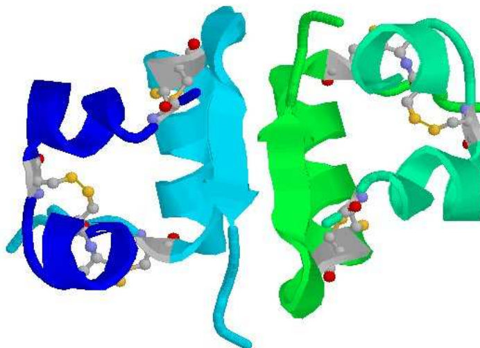
Figura 3.6 Duas moléculas de insulina com as pontes dissulfeto em destaque. (Construída a partir das coordenadas 1GUJ, disponíveis no PDB, Protein Data Bank)
