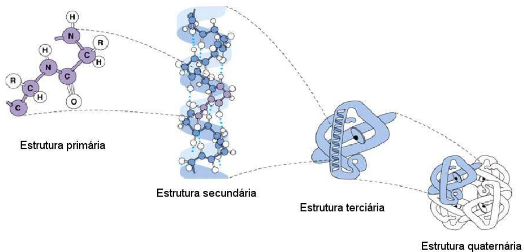
Figura 3.1 Níveis de organização da estrutura molecular de uma proteína.
