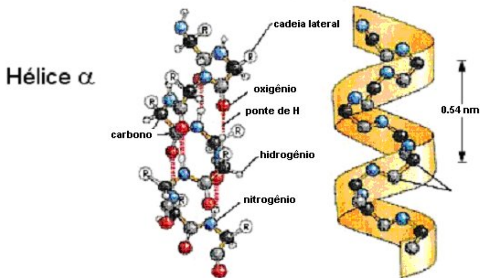
Figura 3.2 Exemplo de uma estrutura do tipo hélice-alfa.
