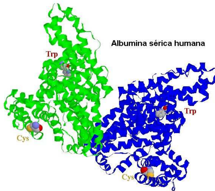
Figura 3.5 Estrutura quaternária da HSA com os resíduos de cisteína e triptofano em destaque. (Construída a partir das coordenadas 1BM0, disponíveis no PDB, Protein Data Bank)
