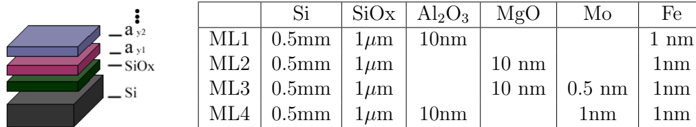
Figura 3.6: Estrutura de um substrato multicamada. A camada superior é um filme fino de um metal cataliticamente ativo.
