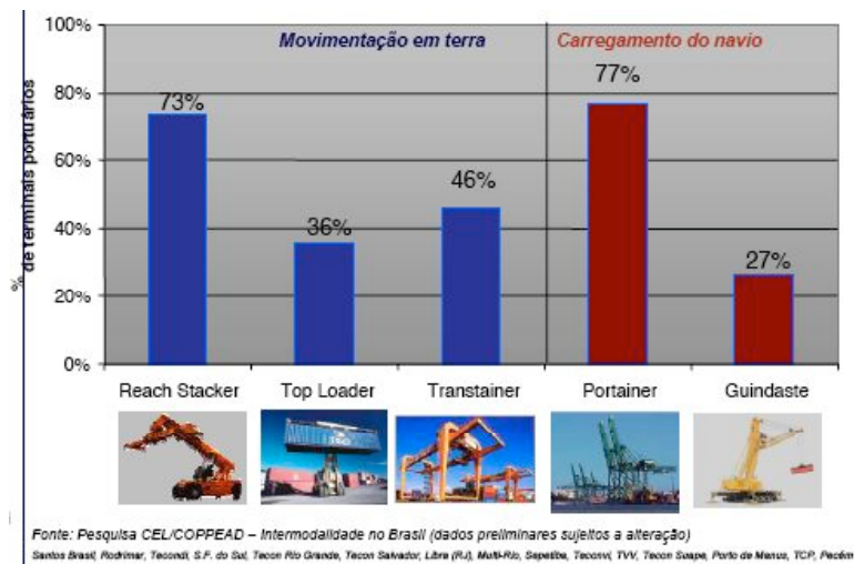
Figura 35 – Percentagem de equipamentos utilizados nos terminais de Contêineres brasileiros
