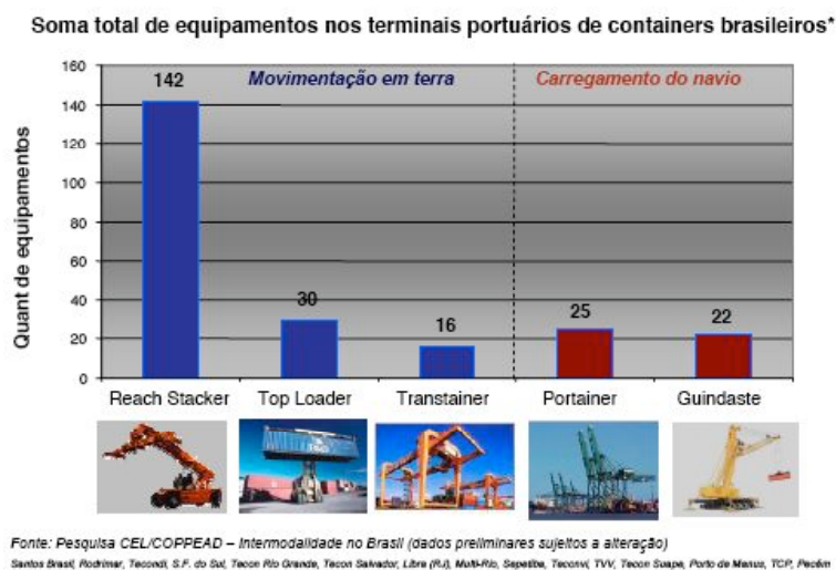
Figura 34 – Soma de equipamentos utilizados nos terminais brasileiros de Contêineres
