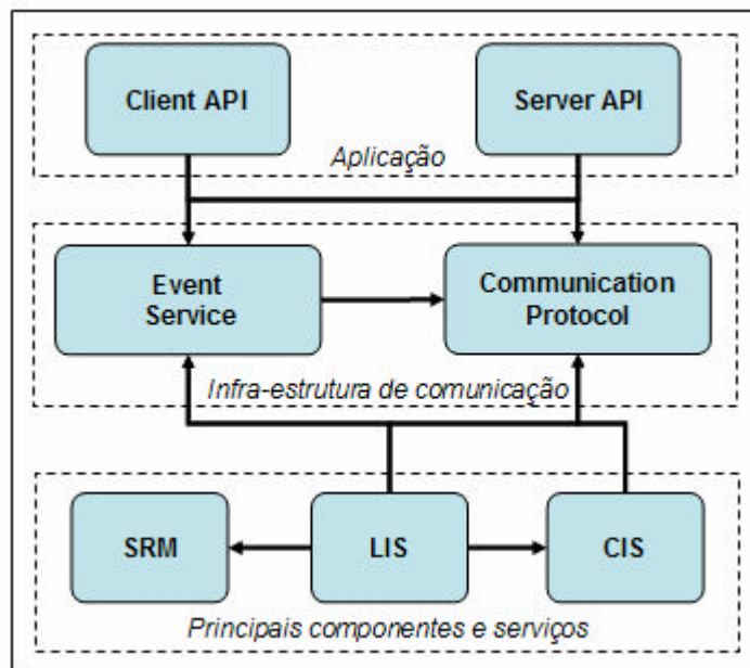
Figura 2. Dependências entre as APIs de MoCA
