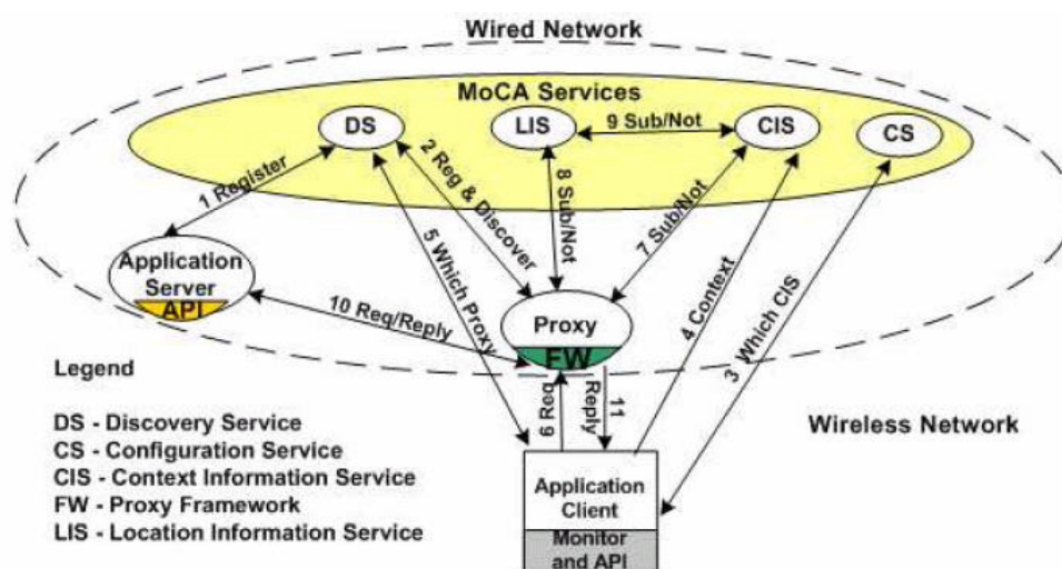
Figura 1. Arquitetura MoCA (Sacramento et al., 2004)
