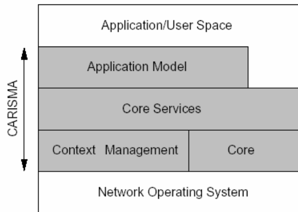
Figura 4. Arquitetura CARISMA (Capra et al., 2003)
