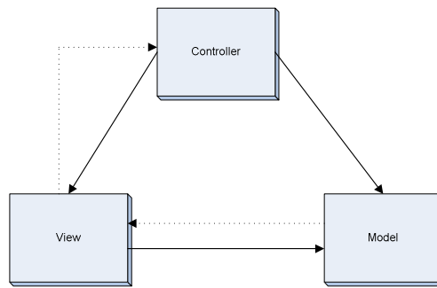
Figura 26: Modelo MVC
