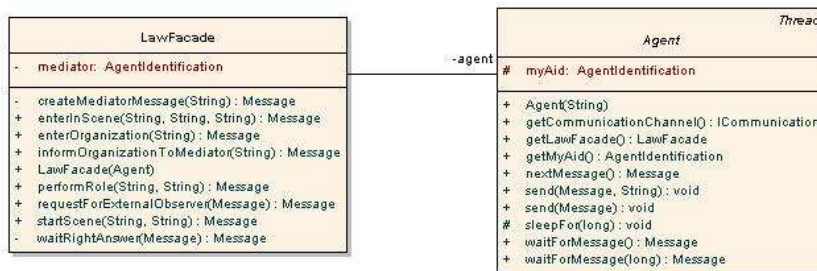
Figura 4.1: Estrutura de Classes de um Agente XMLaw
