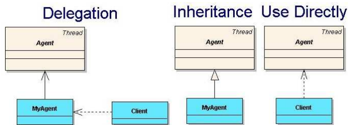
Figura 4.2: Formas de utilização de um agente XMLaw
