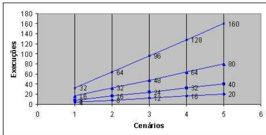
Figura 4.3: Quantidade de Execuções por Cenário de Teste
