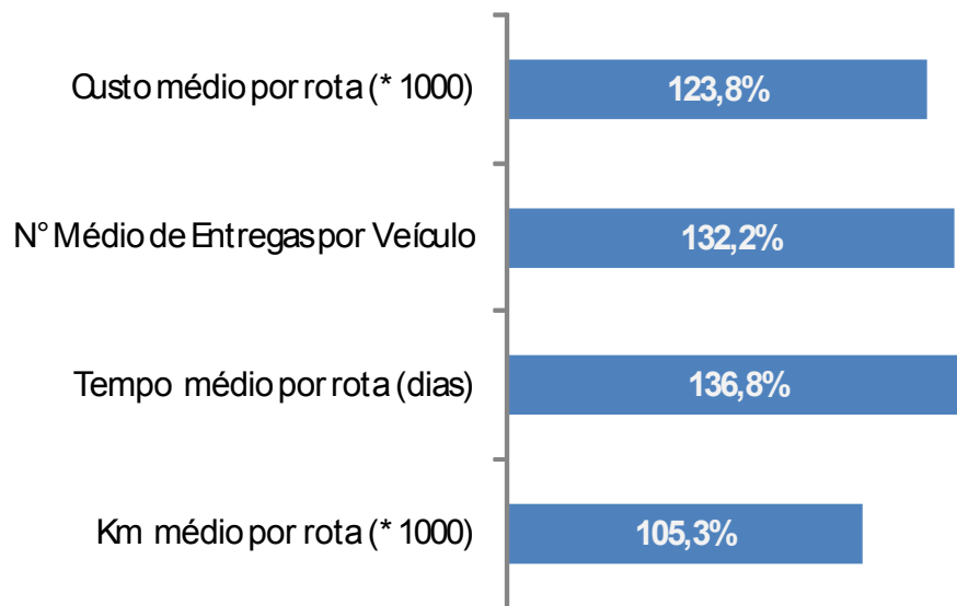
Gráfico 13 – Comparativo percentual entre os indicadores do modelo de Clarke e Wright e de Rotas Fixas
