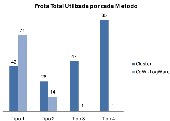
Gráfico 10 – Total de veículos utilizados nos 10 dias analisados
