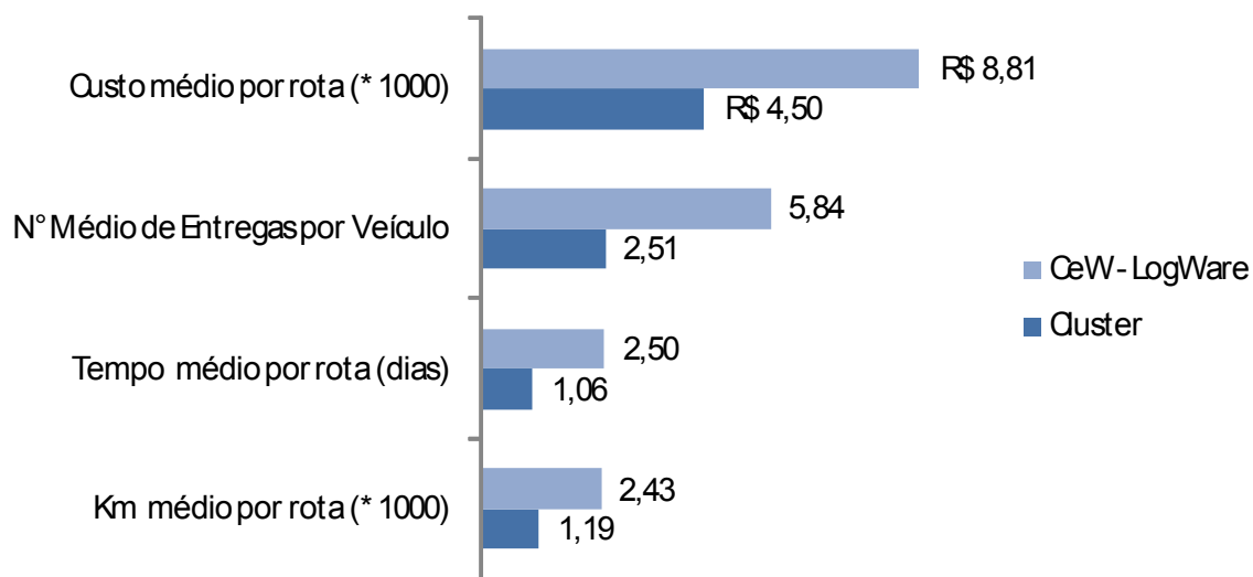
Gráfico 12 – Dados comparativos de desempenho de cada um dos métodos
