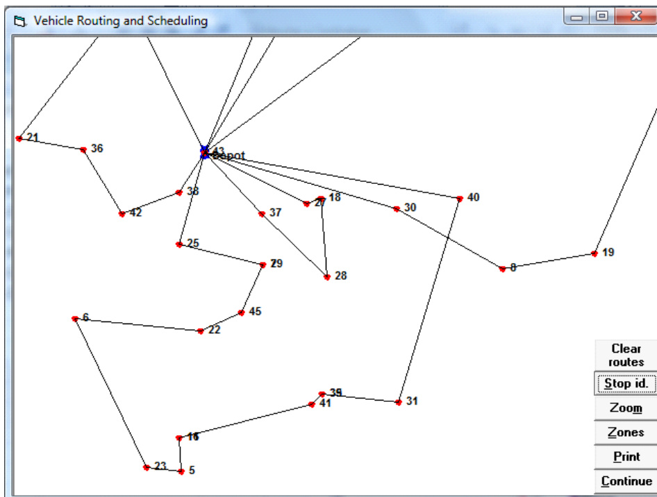
Figura 20 - Rotas geradas pelo Router para o dia 08 de outubro
