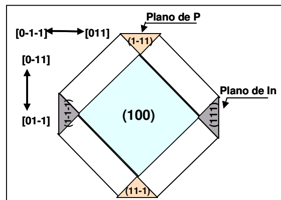
Figura 7.8. Esquema mostrando o substrato de InP ressaltando seus planos e direções cristalinas.
