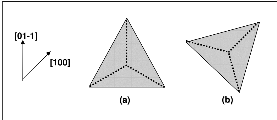
Figura 7.1. Direções de alinhamento da ponta Berkovich nas medidas realizadas. Em (a) uma das quinas da ponta está alinhada com a direção [01-1] do InP e em (b) a ponta está alinhada com a direção [100] .
