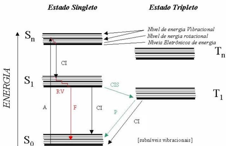
Figura 2.3 – Diagrama de Jablonski modificado. (A) absorção de um fóton, ( S_0 ) estado fundamental de singlete, ( S_n ) estado excitado de singlete, ( S_1 ) primeiro estado excitado de singlete, (RV) relaxação vibracional, (CI) conversão interna, (CIS) cruzamento intersistemas, ( T_n ) estado excitado de tripleto.
