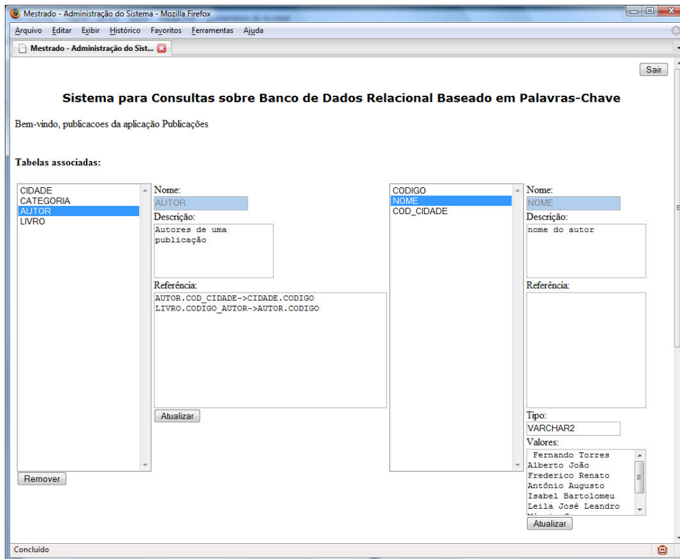
Figura 10: Página de Edição da Aplicação Publicações
