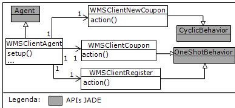
Figura 20. Reengenharia do Módulo Cliente de WMS usando ESSMA
