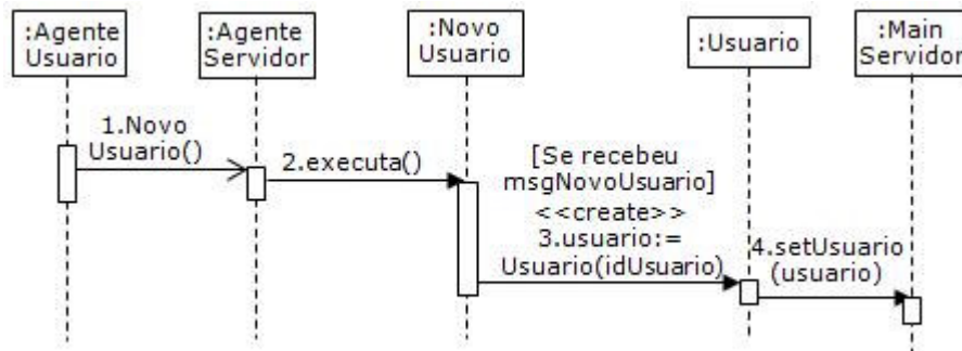
Figura 17. Cenário de Criação do Usuário em VL
