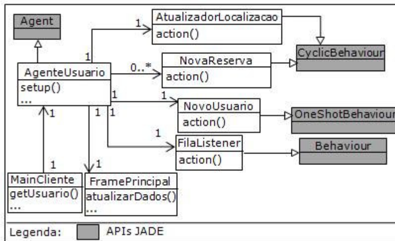
Figura 15. Reengenharia do Módulo Cliente de VL usando ESSMA
