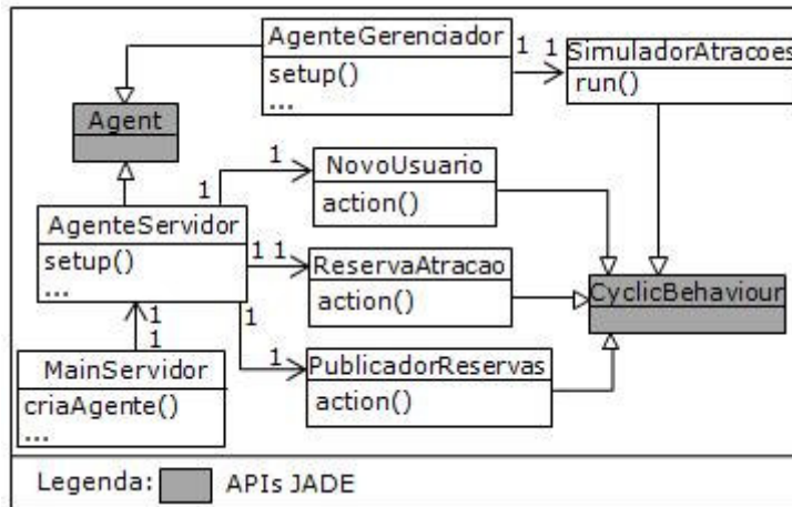
Figura 16. Reengenharia do Módulo Servidor de VL usando ESSMA
