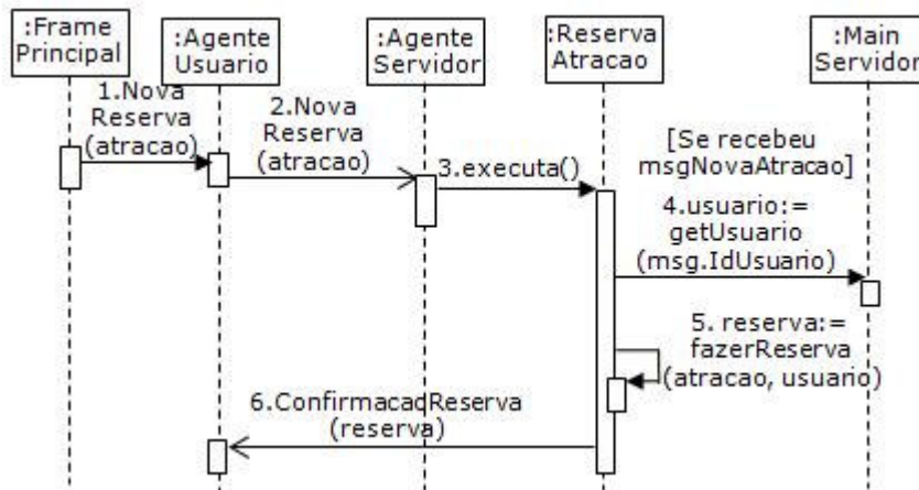
Figura 18. Cenário de Solicitação de uma Reserva em VL
