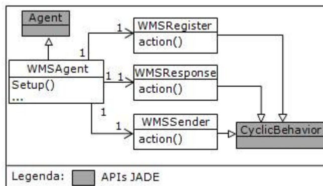
Figura 19. Reengenharia do Módulo Servidor de WMS usando ESSMA
