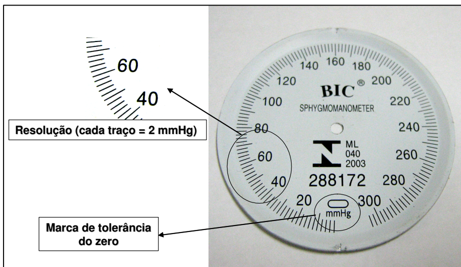
Figura 5 – Escala de leitura do esfigmomanômetro mecânico.
