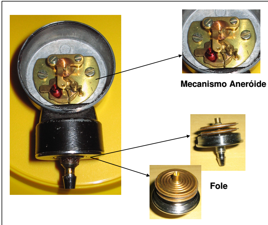
Figura 12 – partes internas do mecanismo aneróide do esfigmomanômetro.
