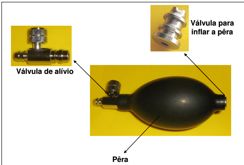
Figura 9 – Ilustração dos componentes do mecanismo para inflar o manguito.
