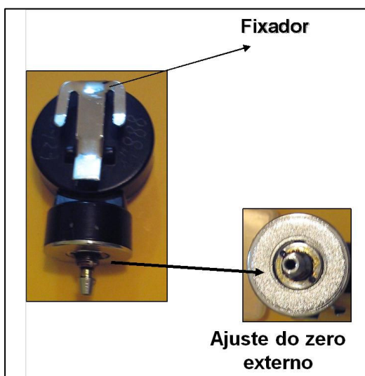
Figura 6 – Ilustração da parte traseira do manômetro.
