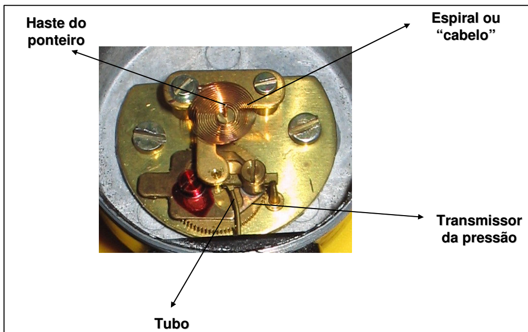
Figura 11 – Mecanismo aneróide.
