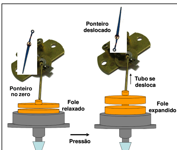
Figura 13 – Mecanismo do esfigmomanômetro mecânico aneróide.
