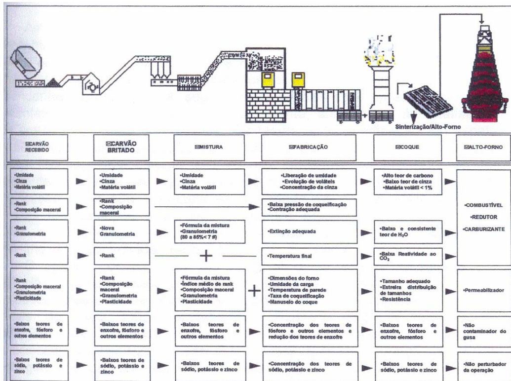
Figura 3: Levantamento de parâmetros metalúrgicos para carvão aplicado à fabricação de coque de alto-forno.
