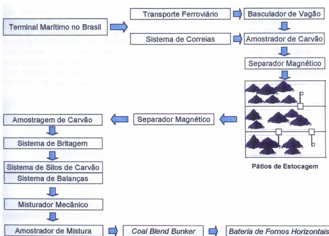
Figura 1: Fluxo do carvão mineral em usina siderúrgica a coque.
