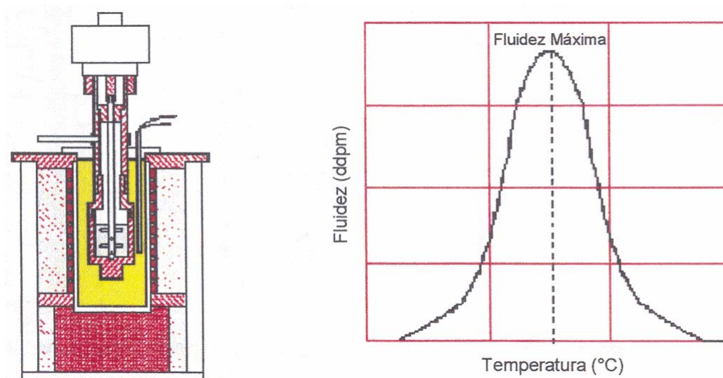
Figura 4: Plastômetro de Gieseler e curva de variação da fluidez com a elevação da temperatura da amostra de carvão.
