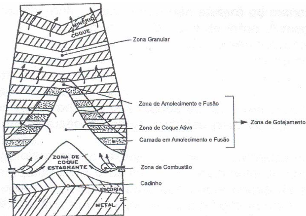
Figura 2: Estrutura interna do alto-forno e suas principais zonas.
