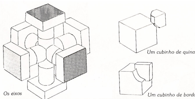
Figura 26: O mecanismo interno do Cubo Mágico (TAYLOR, 1981, p. 5).
