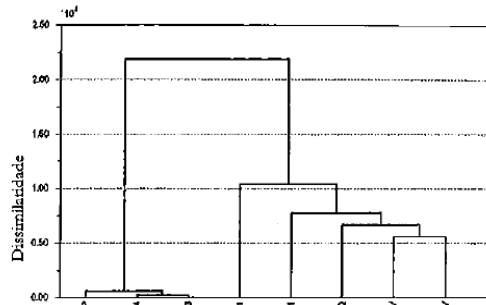
Figura 4 -- Dendograma.
