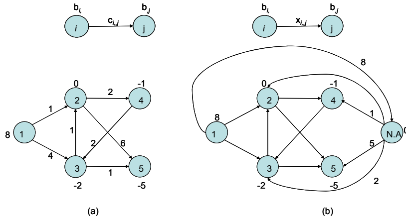
Figura 3.5 - Encontrando uma solução inicial através de um nó artificial.
