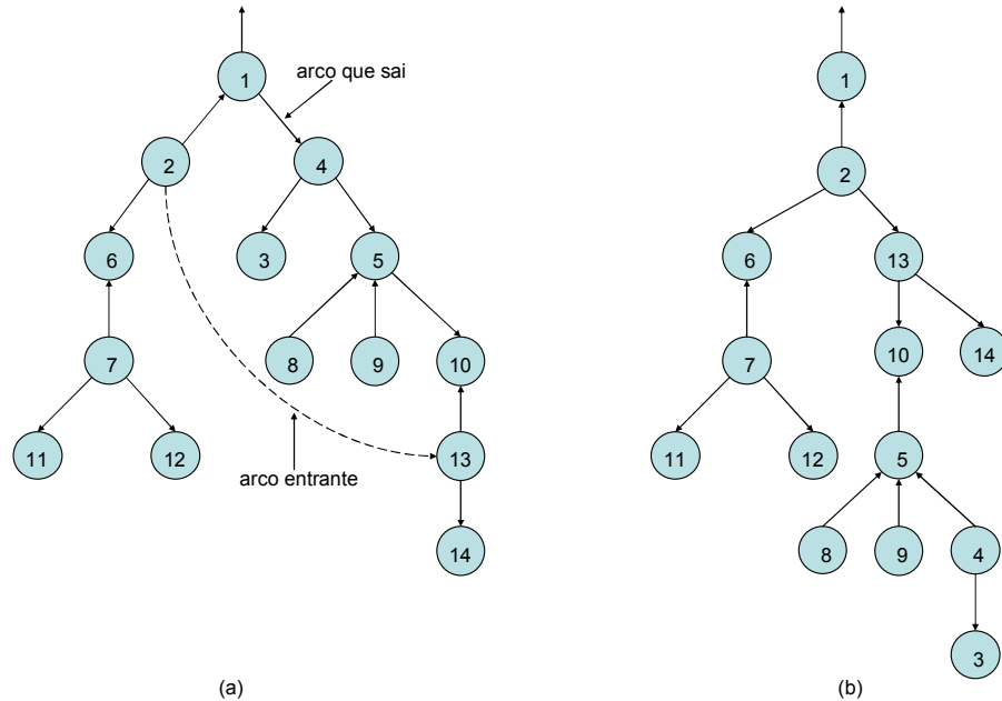
Figura 3.12 - Atualização dos índices da árvore
