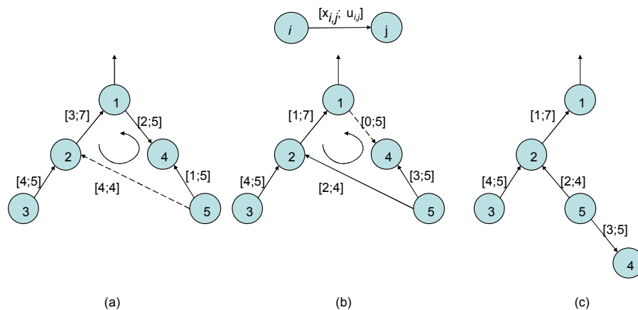
Figura 3.11 - Exemplo de pivoteamento, entrada do arco (5,2) e saída do arco (1,4) .
