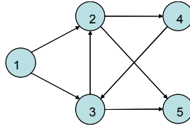
Figura 3.2 – Encontrando a matriz de incidência nó-arco
