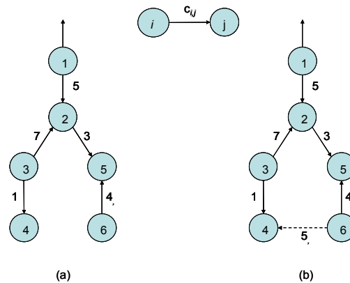
Figura 3.8 - (a) Exemplo de árvore geradora e (b) ciclo formado pela inclusão do arco (6,4).
