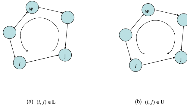
Figura 3.10 - Direção do fluxo ao longo do ciclo de pivoteamento.
