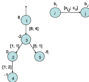
Figura 3.7- Solução factível básica.
