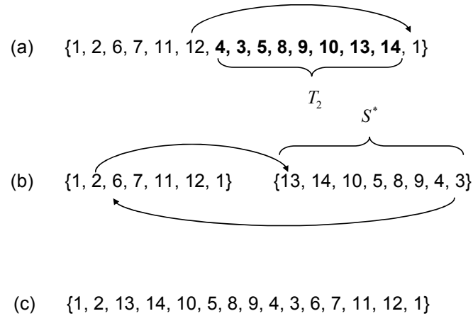
Figura 3.13 – Exemplo: dinâmica de atualização dos índices
