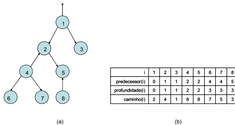
Figura 3.9 - Exemplo de árvore geradora e índices associados
