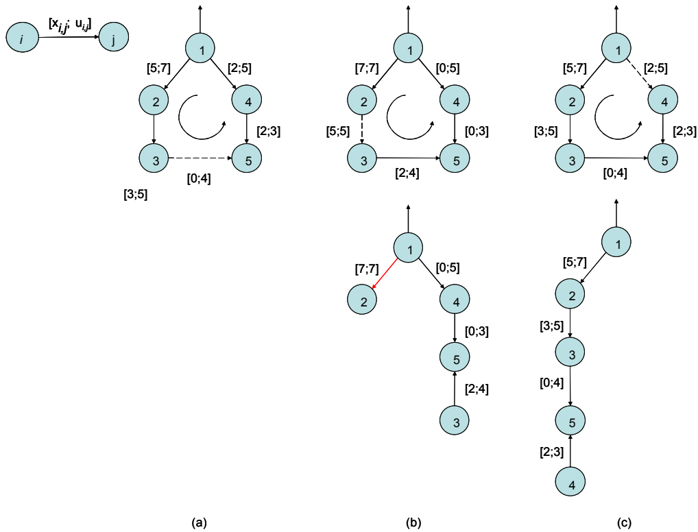
Figura 3.14- Árvores fortemente factíveis, regra de seleção do arco que sai da base.
