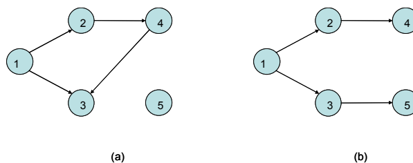
Figura 3.3 - conjuntos de arcos (a), linearmente dependentes, e (b), independentes.
