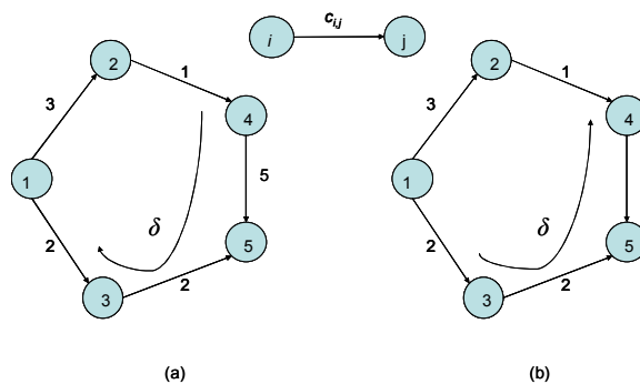
Figura 3.1 - Ciclo composto unicamente por arcos livres.
