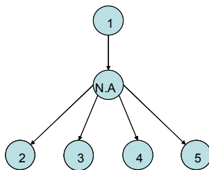
Figura 3.6 - Solução inicial, exemplo.
