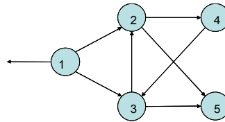
Figura 3.4 - Entrada da Variável Artificial
