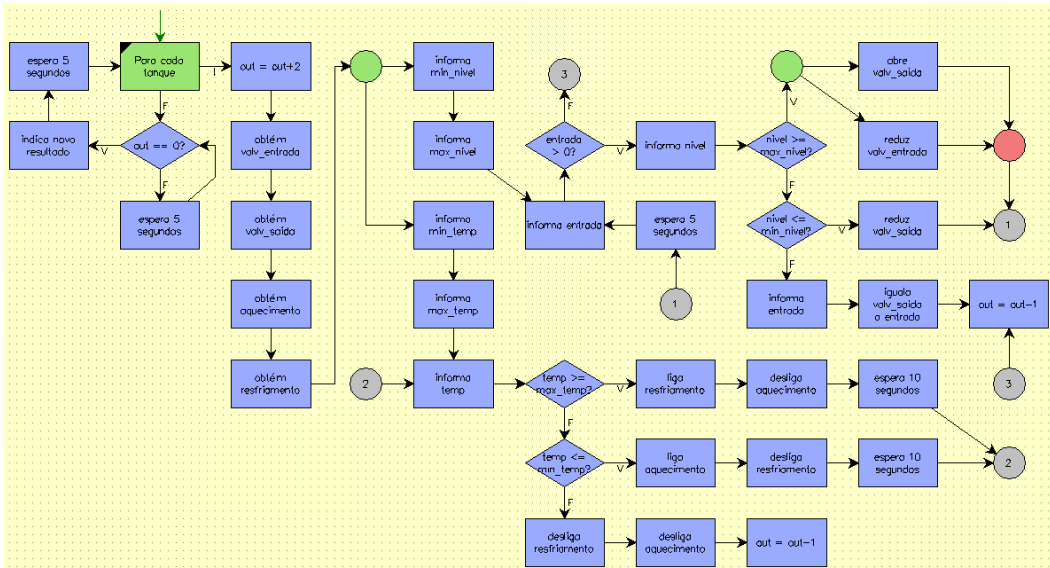
Figura 5.2: Fluxo de controle de temperatura e nível de tanques.
