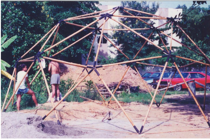
Fig. 11 - Geodésica de bambu desenvolvida no LOTDP.
