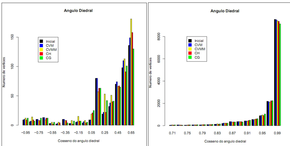
Figura 5.8: Ângulo diedral sobre as arestas do modelo nas deformações apresentadas na figura 5.5.
