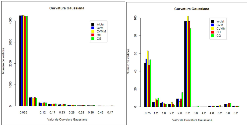
Figura 5.6: Curvatura Gaussiana das deformações da figura 5.5.
