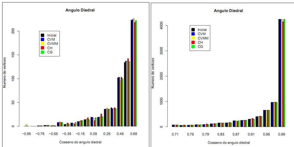
Figura 5.11: Ângulo diedral sobre as arestas do modelo.
