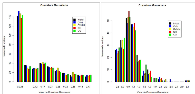
Figura 5.16: Curvatura Gaussiana nos pontos das deformações obtidas na figura 5.15.
