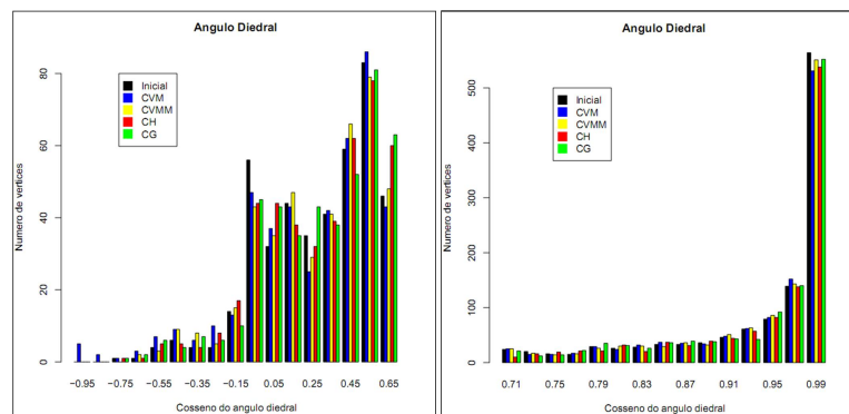
Figura 5.20: Ângulo diedral sobre as arestas nas deformações obtidas na figura 5.18.
