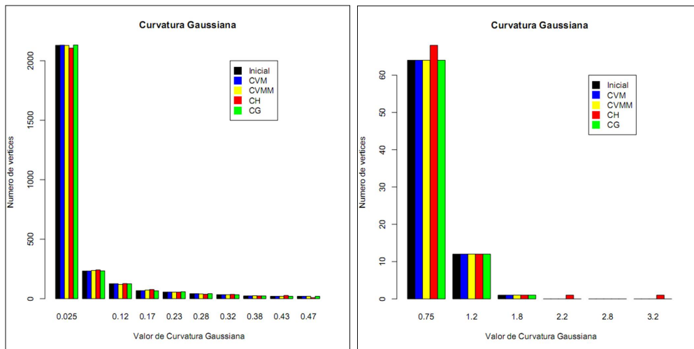
Figura 5.10: Curvatura Gaussiana nos pontos do modelo.
