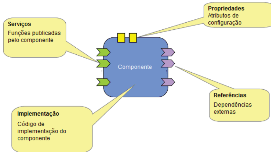
Figura 5.1: Modelo de Componentes SCA
