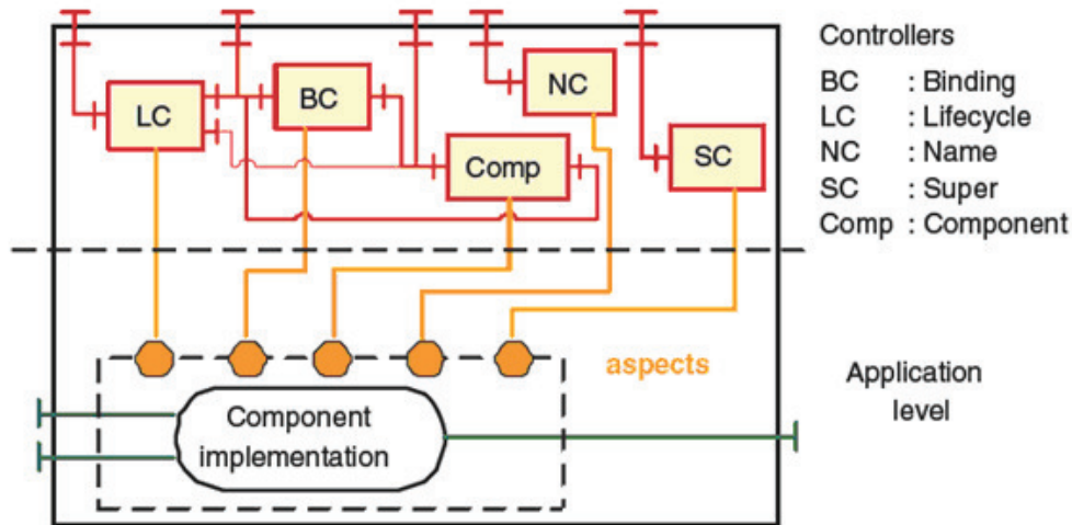
Figura 5.3: AOKell
