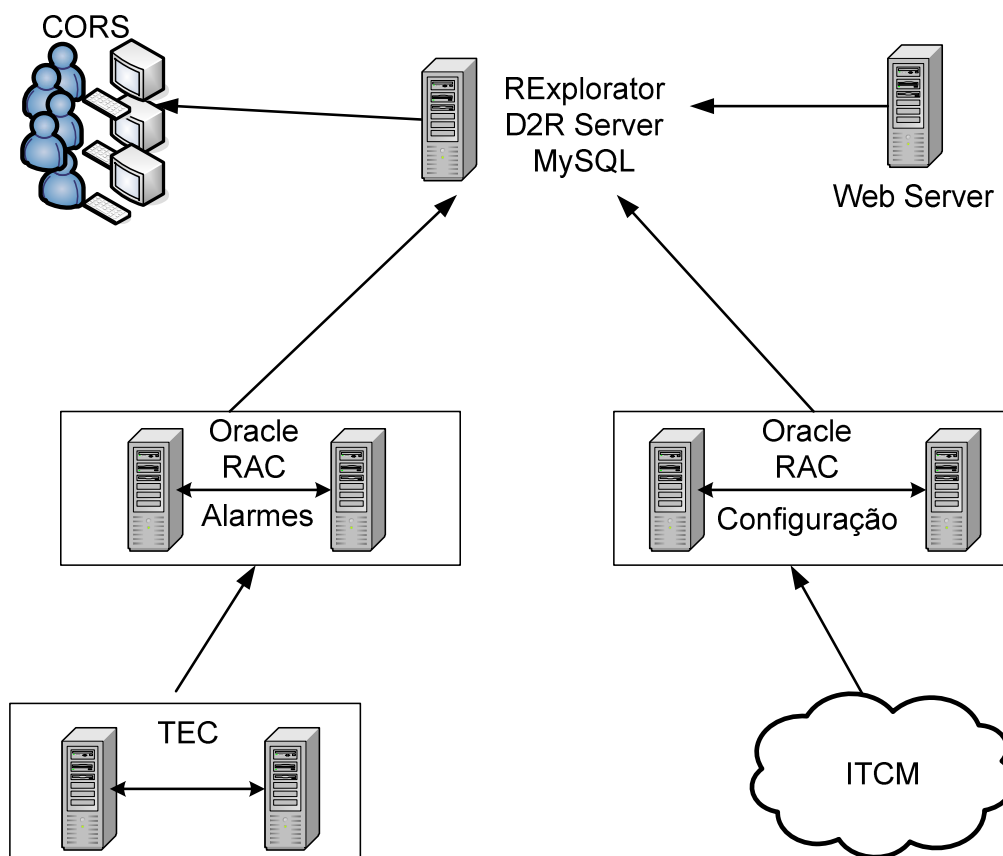
Figura 29 – Arquitetura Física do Ambiente Piloto.
