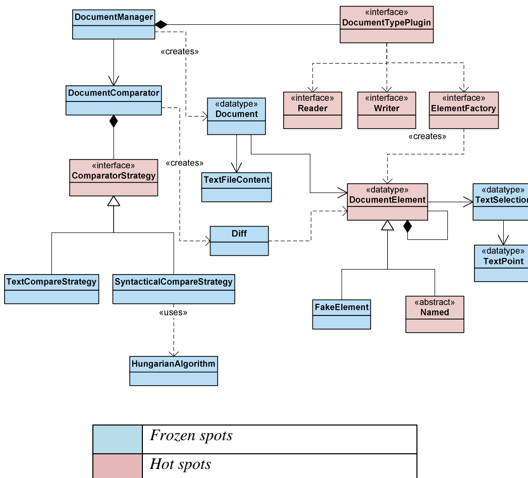
Figura 27 – Diagrama de classes da arquitetura do DMF.
