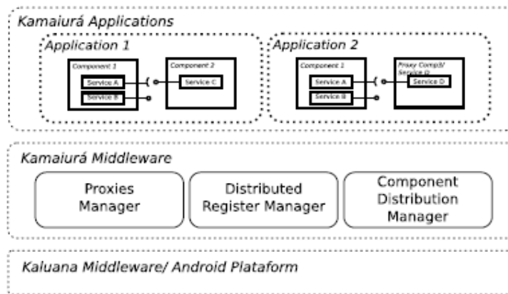
Figura 28. Arquitetura do Kamaiurá sobre o middleware Kaluana
