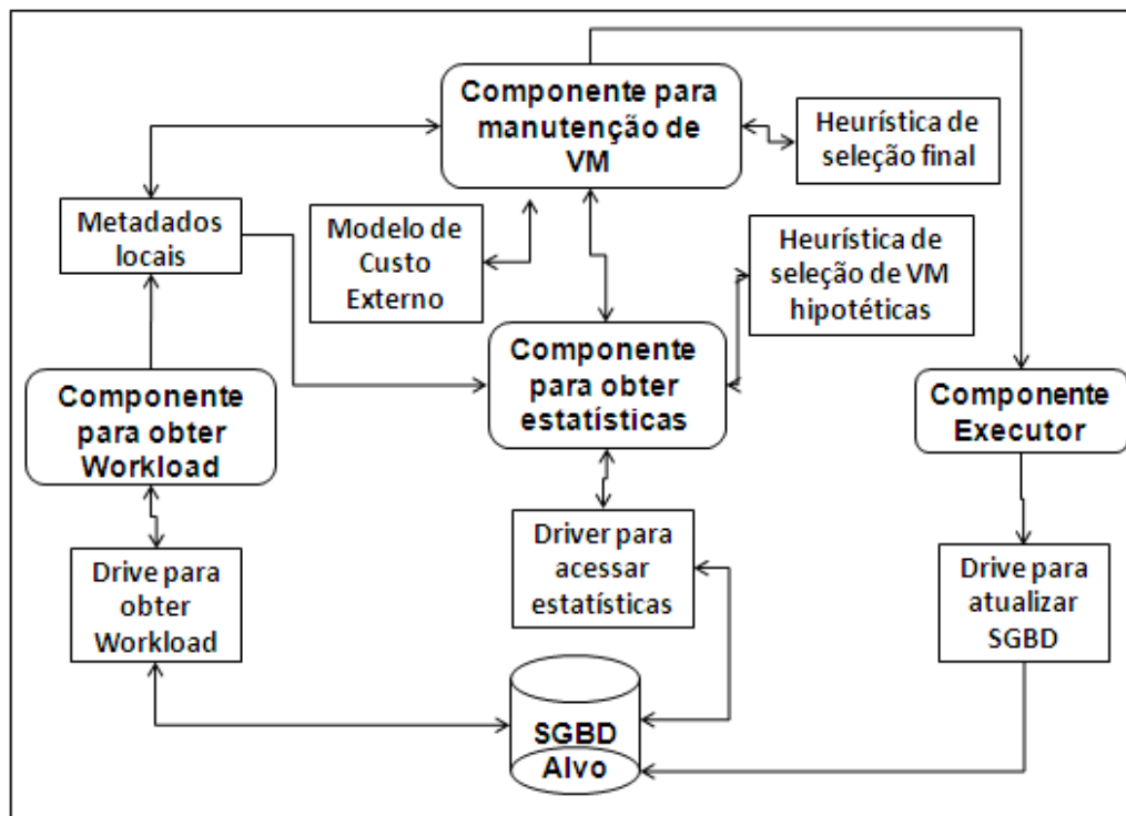
Figura 7 - Arquitetura para gerência de Visão Materializada
