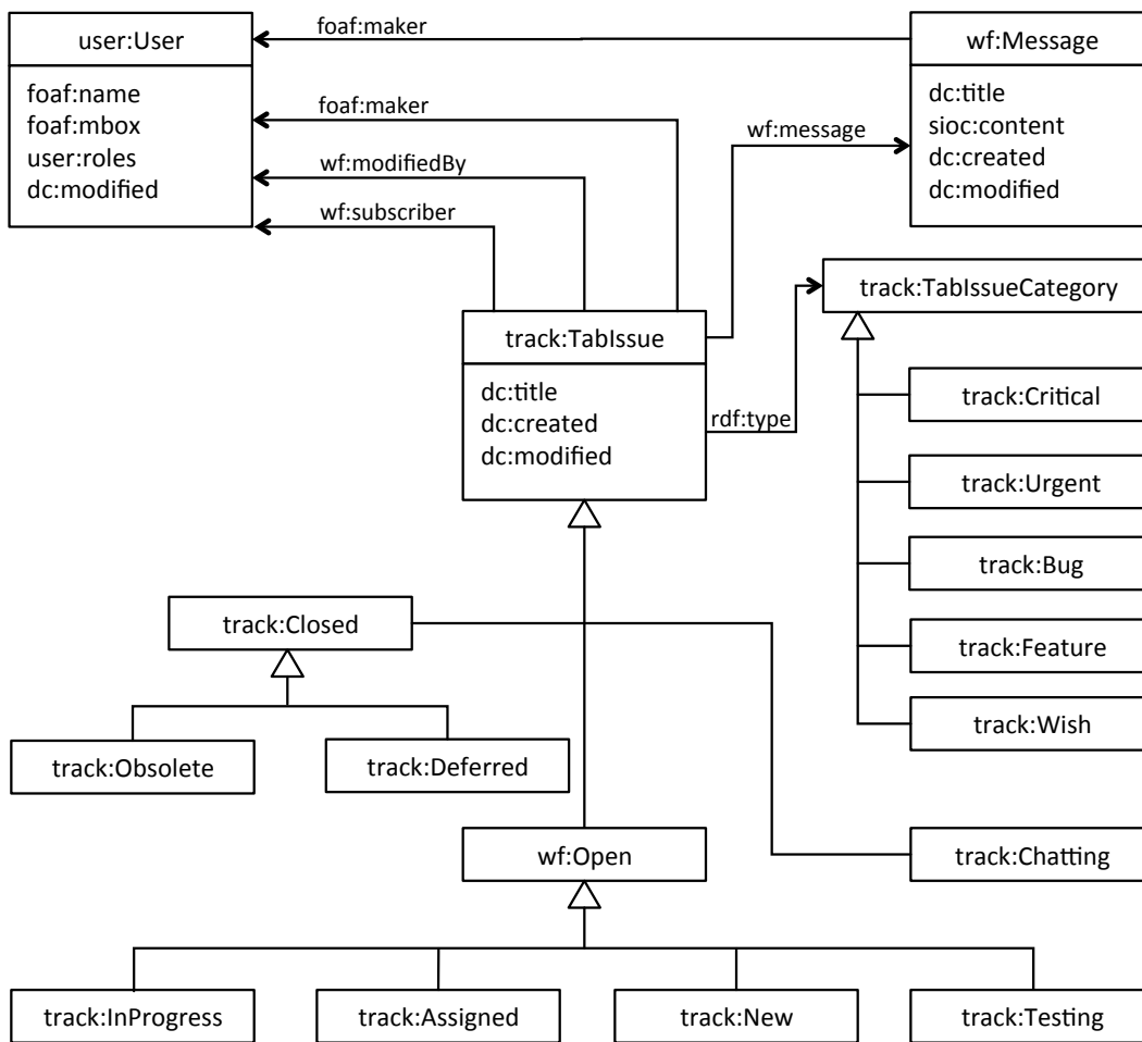
Figura 79 – Ontologia da aplicação Semantic Issue Tracker
