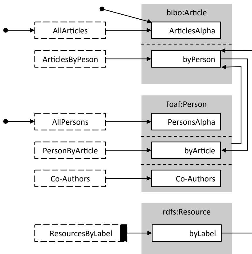
Figura 72 – Esquema de contextos da aplicação “Lattes”
