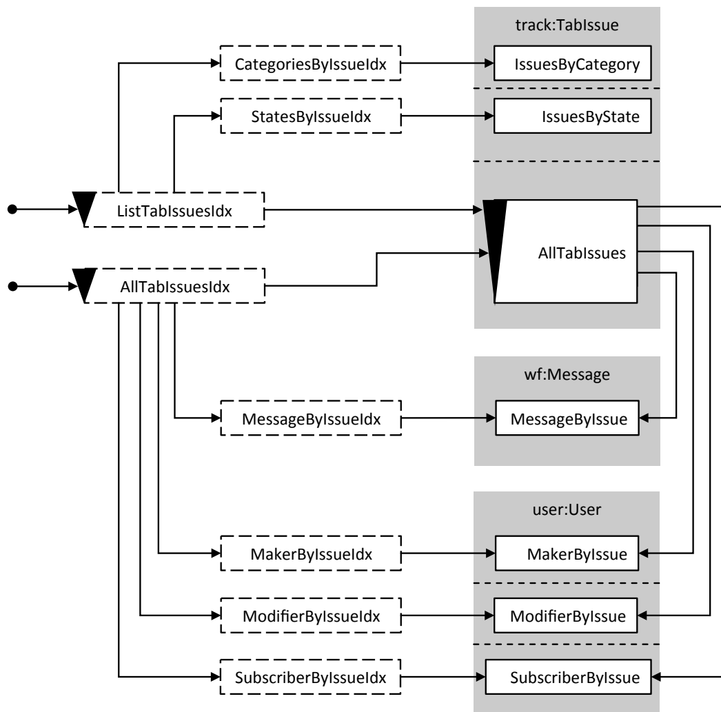
Figura 80 – Esquema de contextos da aplic. Semantic Issue Tracker
