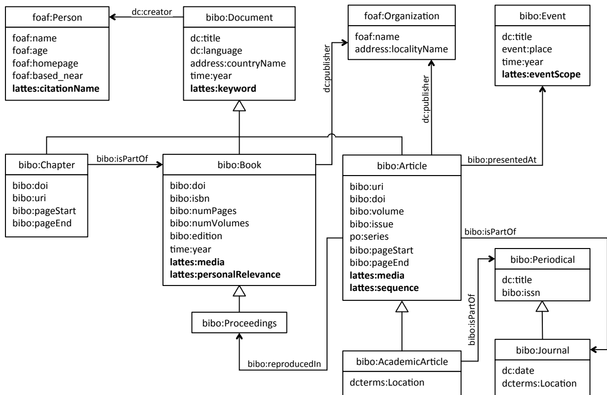
Figura 71 – Ontologia de domínio da aplicação “Lattes”
