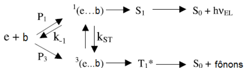
Figura 2.9 - Esquema do processo de eletroluminescência para dispositivos OLEDs baseados em moléculas pequenas. Modificado de [21].
