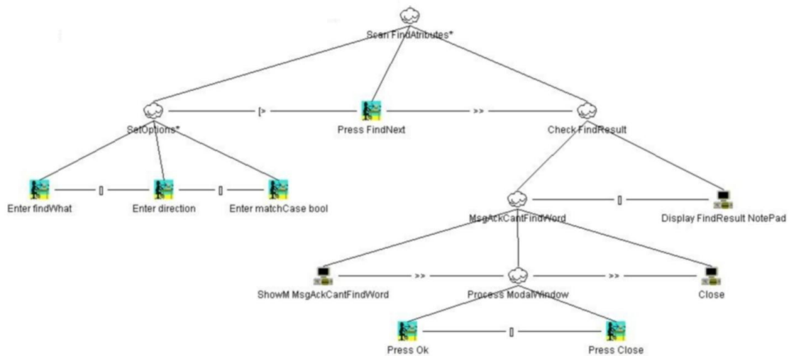
Figura 20 - Diagrama do CTT.
