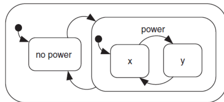
Figura 39 - Estados simples com XOR meta-state.
