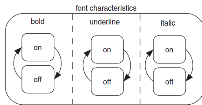
Figura 40 - Estado concorrente com AND meta-state.
