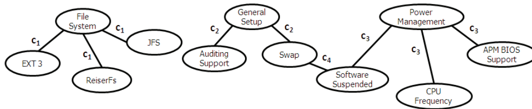
Figura 3.6: Grafo de dependências.
