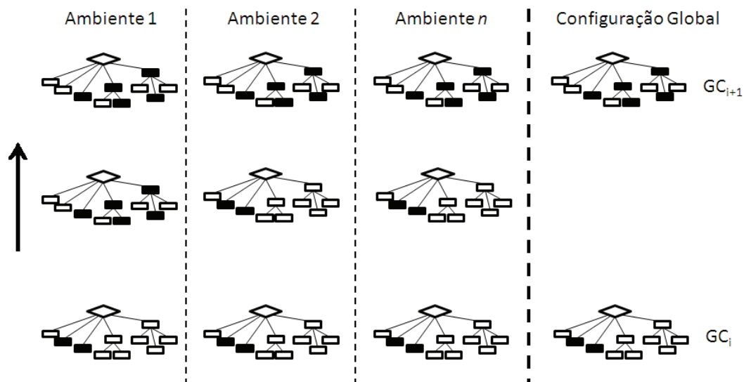
Figura 3.5: Evolução da configuração global de CG_i para CG_{i+1} .
