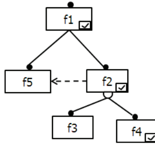
Figura 3.7: Modelo de features para exemplificar filtros de ações de correção.
