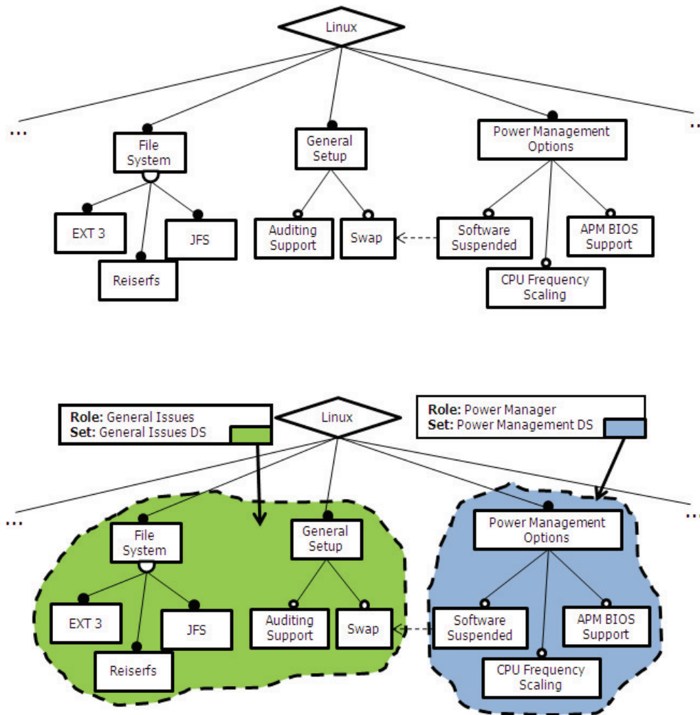
Figura 3.2: Modelo de features reduzido do kernel do Linux.
