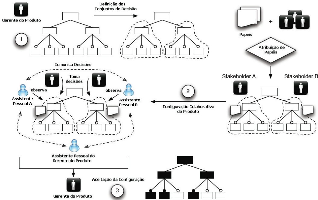
Figura 3.1: Visão geral da proposta de configuração dinâmica e distribuída de produtos.
