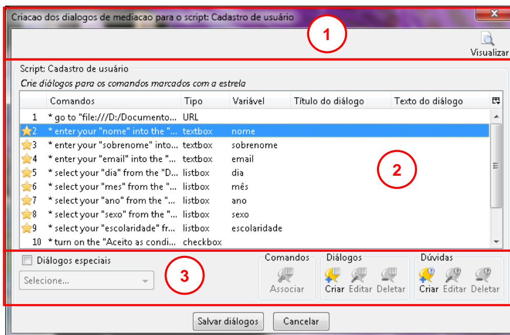
Figura 3.23 – Tela inicial do editor de diálogos
