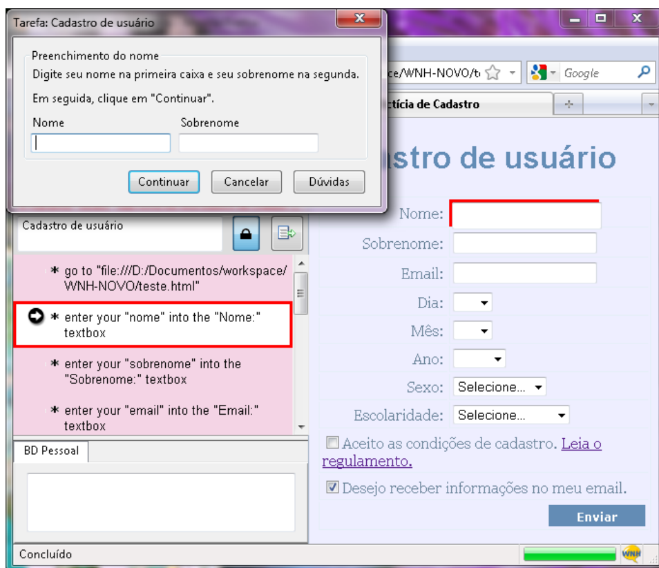
Figura 3.37 – Diálogo em execução no editor de scripts
