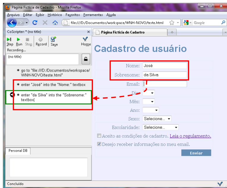
Figura 3.5 – Início da gravação do Script
