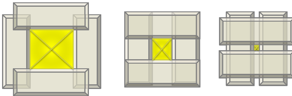
FIGURA 12 – Simulação de tamanhos de campo de radiação com colimador secundário formado por quatro blocos.
