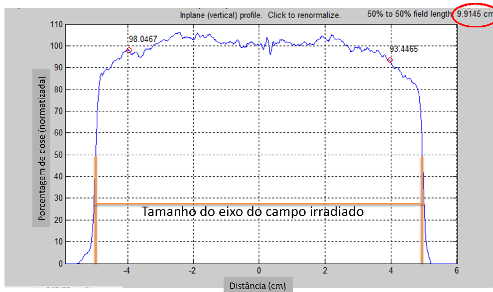
FIGURA 14 – Perfil do feixe utilizado para definição do tamanho de campo a 50% da dose irradiada.
