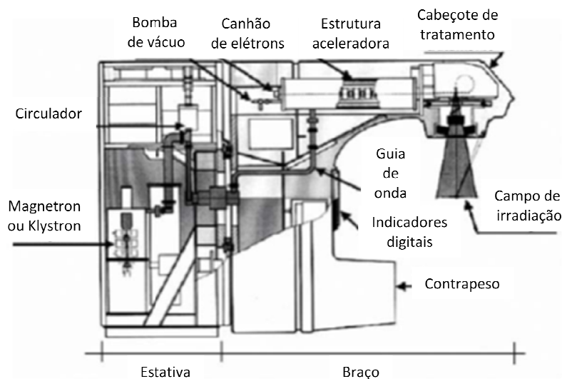
FIGURA 8 – Diagrama de um acelerador linear [19].
