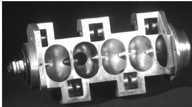
FIGURA 9 - Vista em corte do guia de onda do acelerador linear de 6 MV [18].
