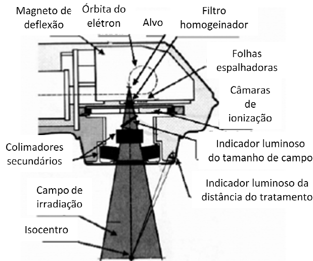
FIGURA 11 - Detalhes dos componentes do cabeçote de um acelerador linear [19].
