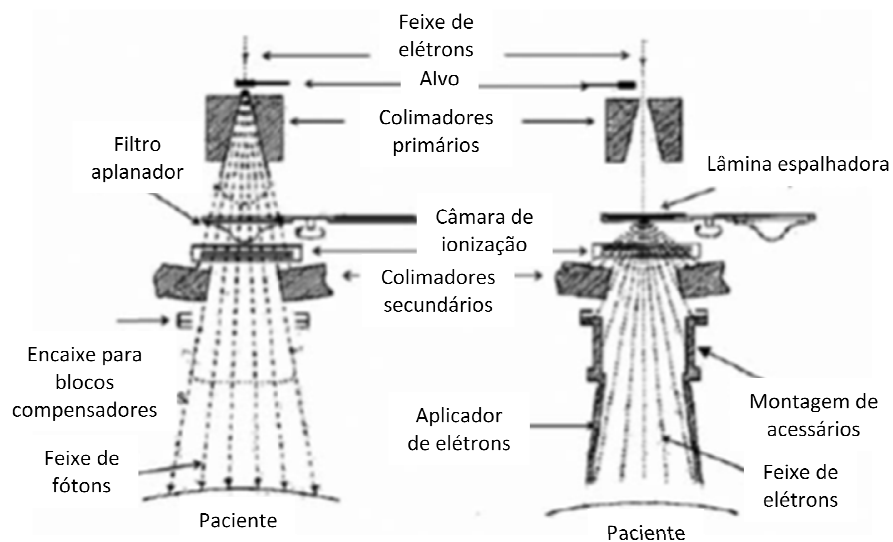
FIGURA 10 - Esquemas do cabeçote de um acelerador para produção de fótons e elétrons [19].
