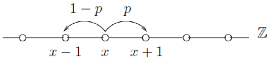
Figura 5.1: Esquema da caminhada aleatória simples.
