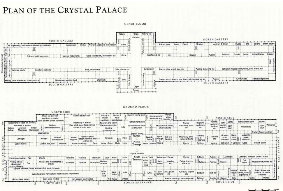
Figura2- Planta baixa do Crystal Palace , 1851, Londres.
