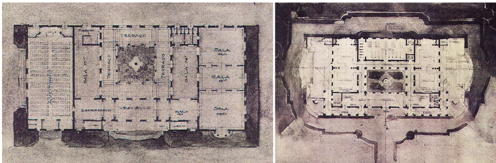
Figura25- Plantas baixas do pavimento principal dos projetos de Nereo Sampaio e Lucio Costa para o pavilhão do Brasil na Exposição da Filadélfia.
