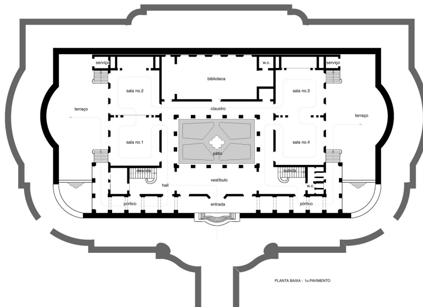
Figura29- Planta baixa - 1o. pavimento - Projeto de Lucio Costa.
