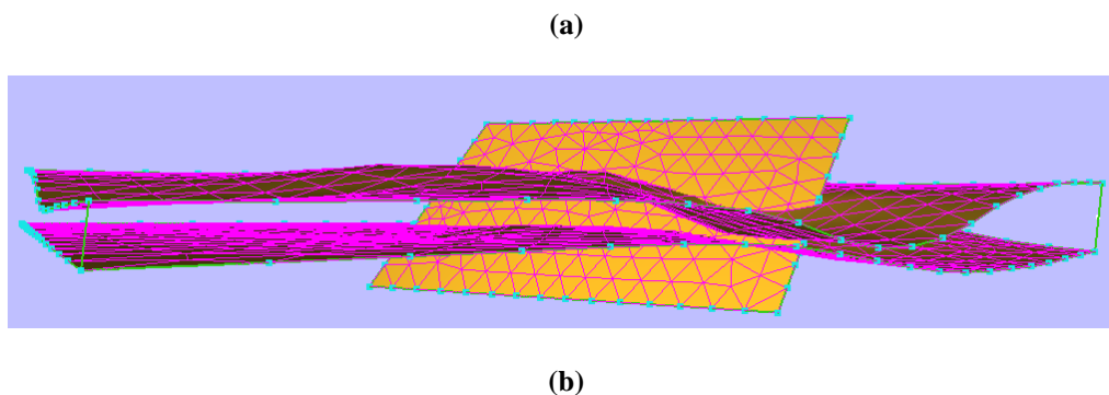
Figura 37: Modelo 20: Interseção de Falha com dois Horizontes
