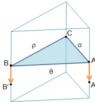
Figura 4: Planos Delimitadores do Triângulo no Algoritmo de MARQUES ET AL. (2010)
