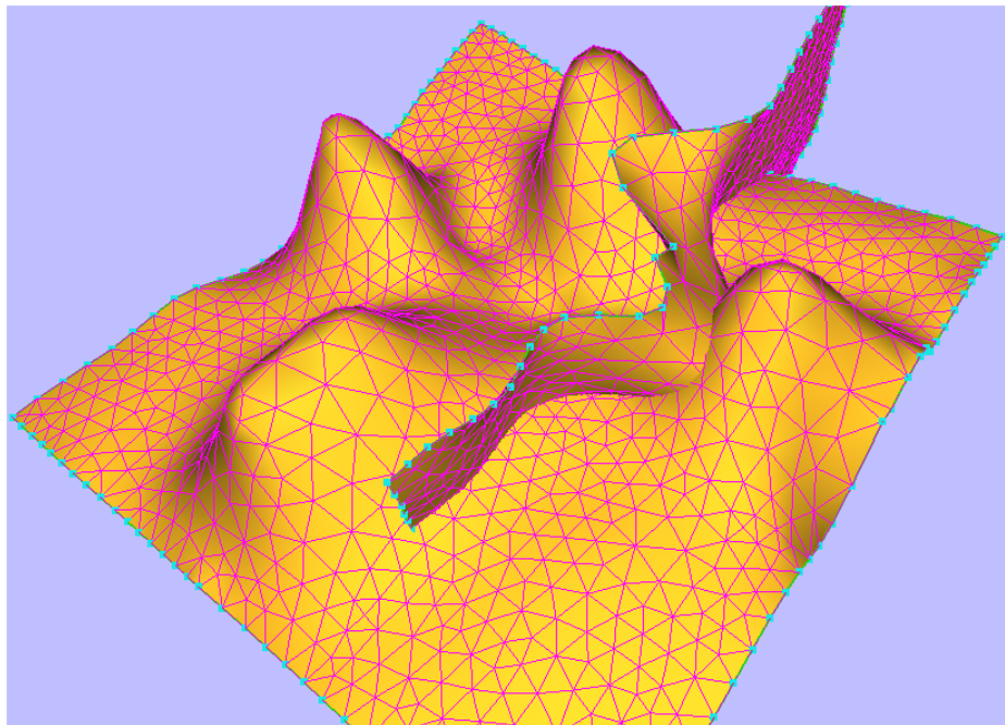
Figura 29: Modelo A: Interseção arbitrária entre superfícies representando domos de sal
