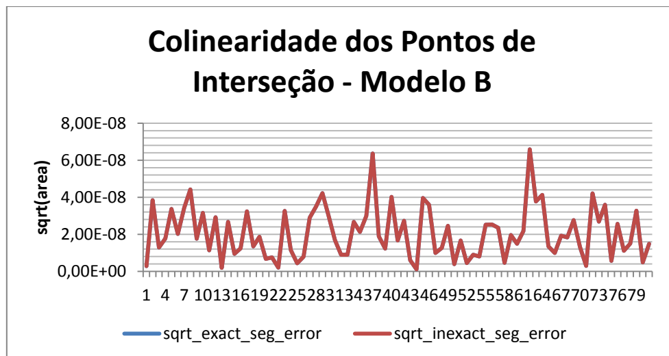
Figura 46: Gráfico do teste de Colinearidade dos Pontos de Interseção do Modelo B
