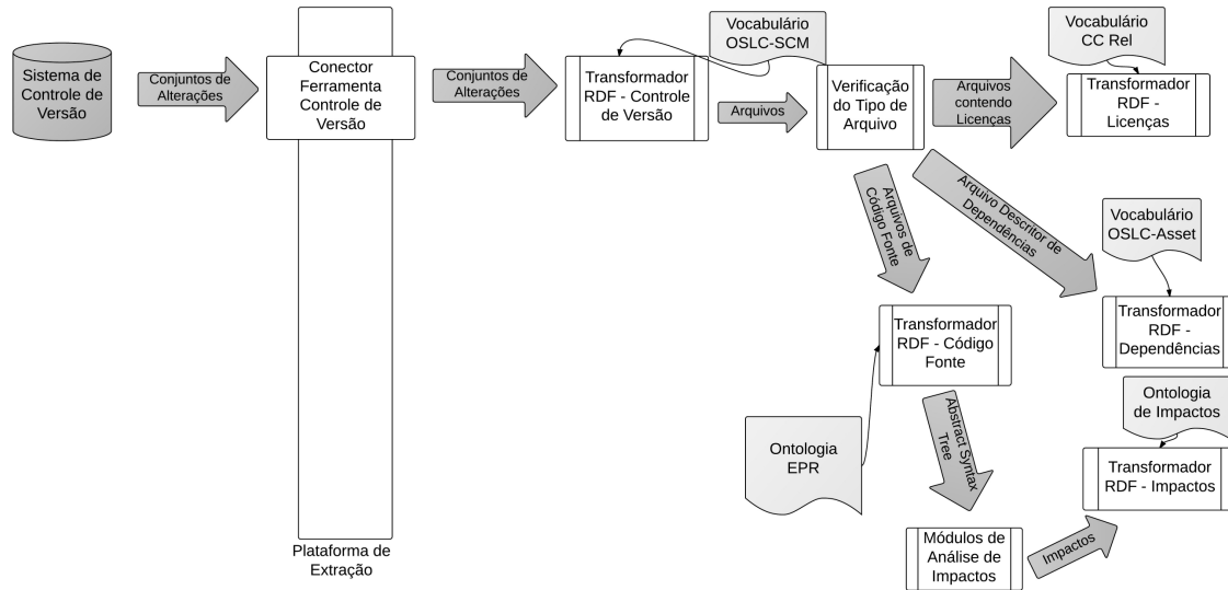
Figura 24 Visão Geral do Processo de Extração de Informações de Ferramentas de Controle de Versão
