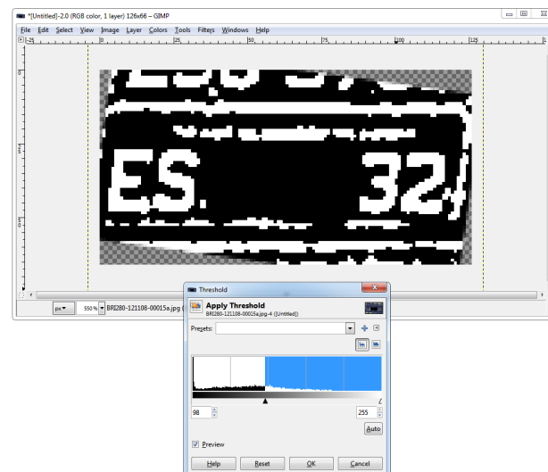
Figura 5.4: Ferramenta Threshold
