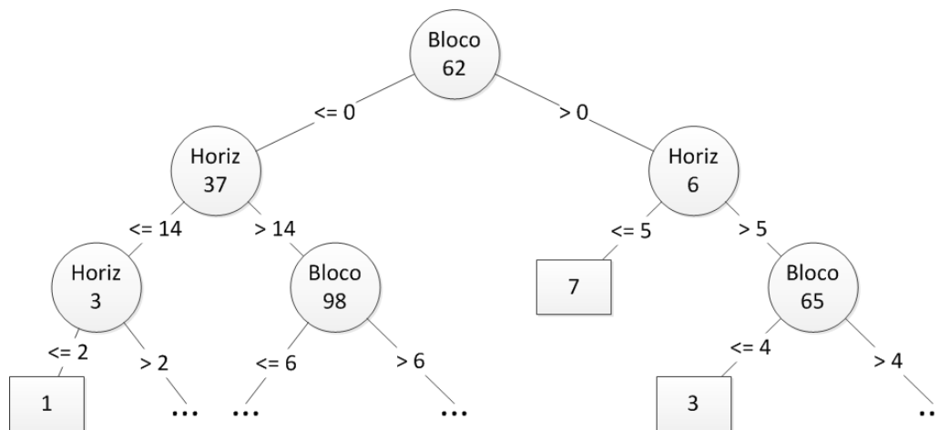
Figura 4.5: Árvore de decisão gerada
