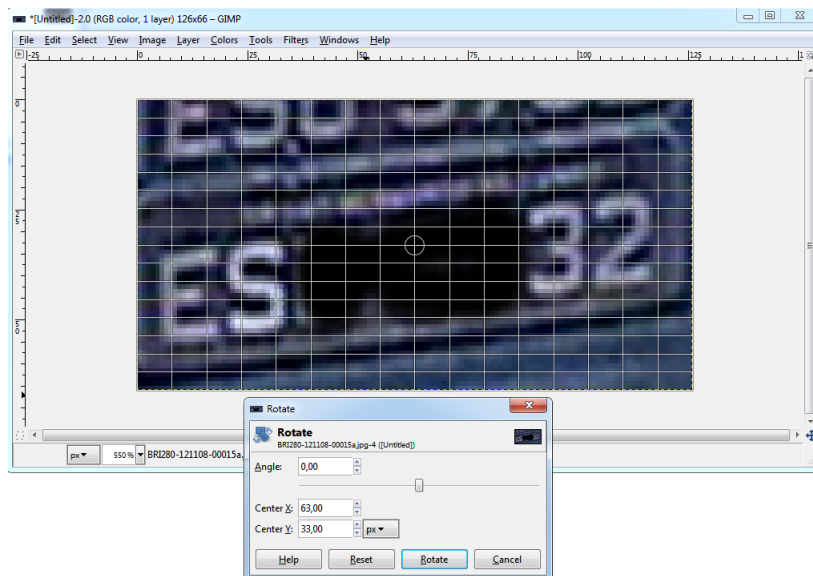
Figura 5.3: Ferramenta Rotate
