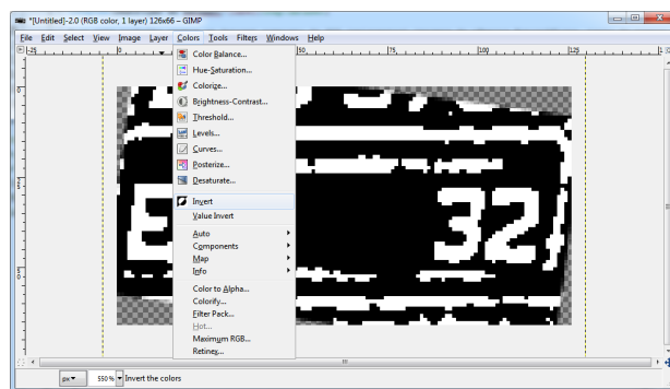
Figura 5.5: Ferramenta Invert
