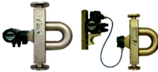
Figura 7 - Medidor coriolis integral e remoto
