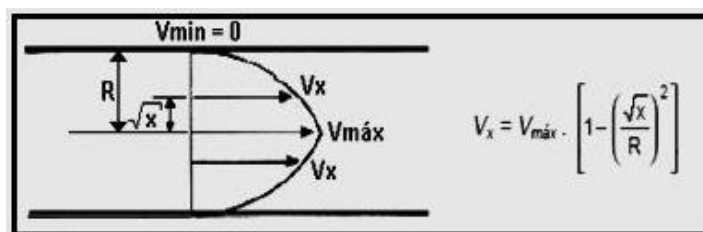
Figura 1 - Perfil de velocidades em regime laminar
