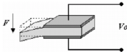
Figura 10 - Efeito Piezoelétrico Direto
