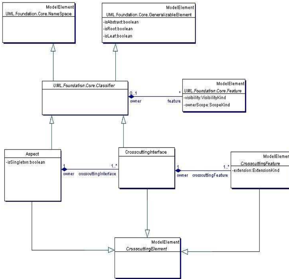
Figura 6.7: Aspect Core: Aspectos
