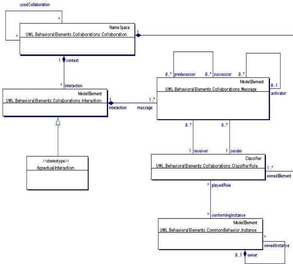
Figura 6.10: Interações aspectuais.
