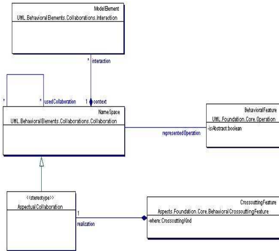
Figura 6.9: Colaborações aspectuais.
