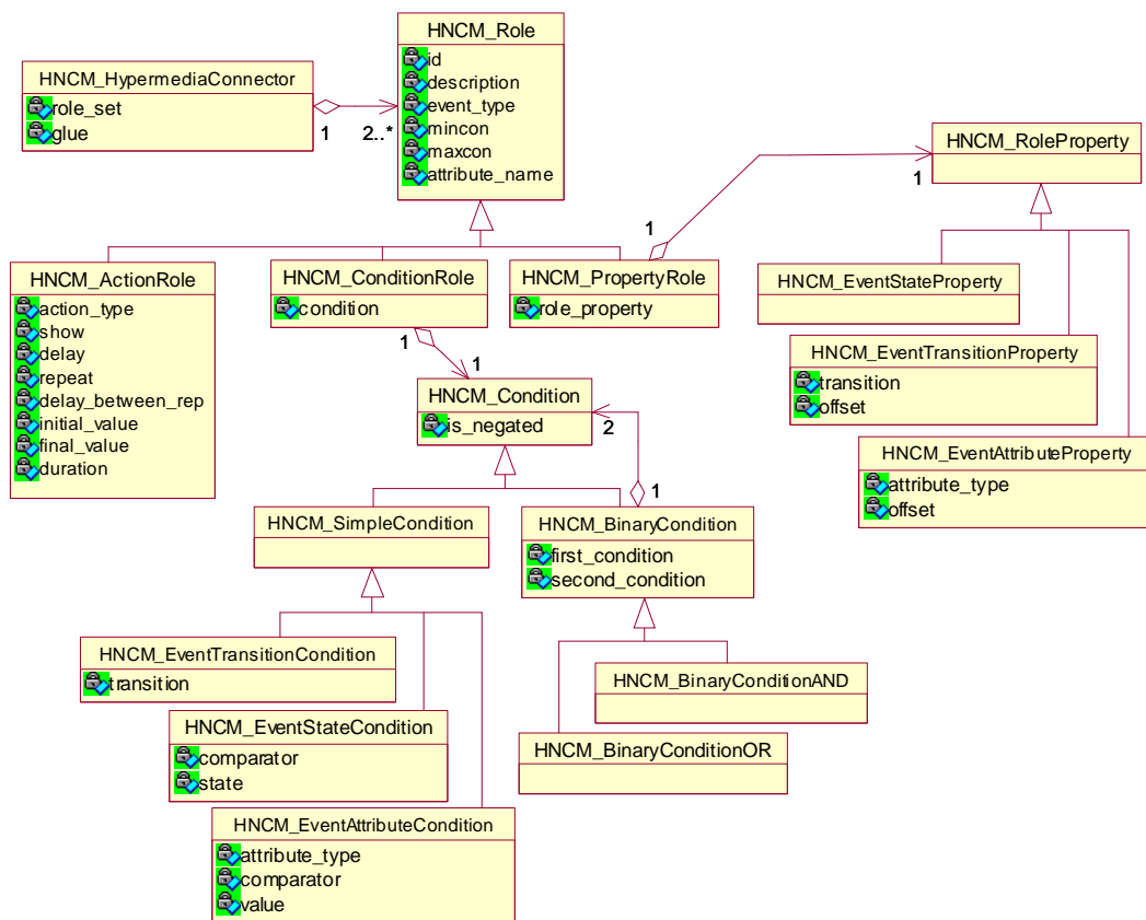
Figura 35. Diagrama de classes para papéis do tipo ação, condição e propriedade
