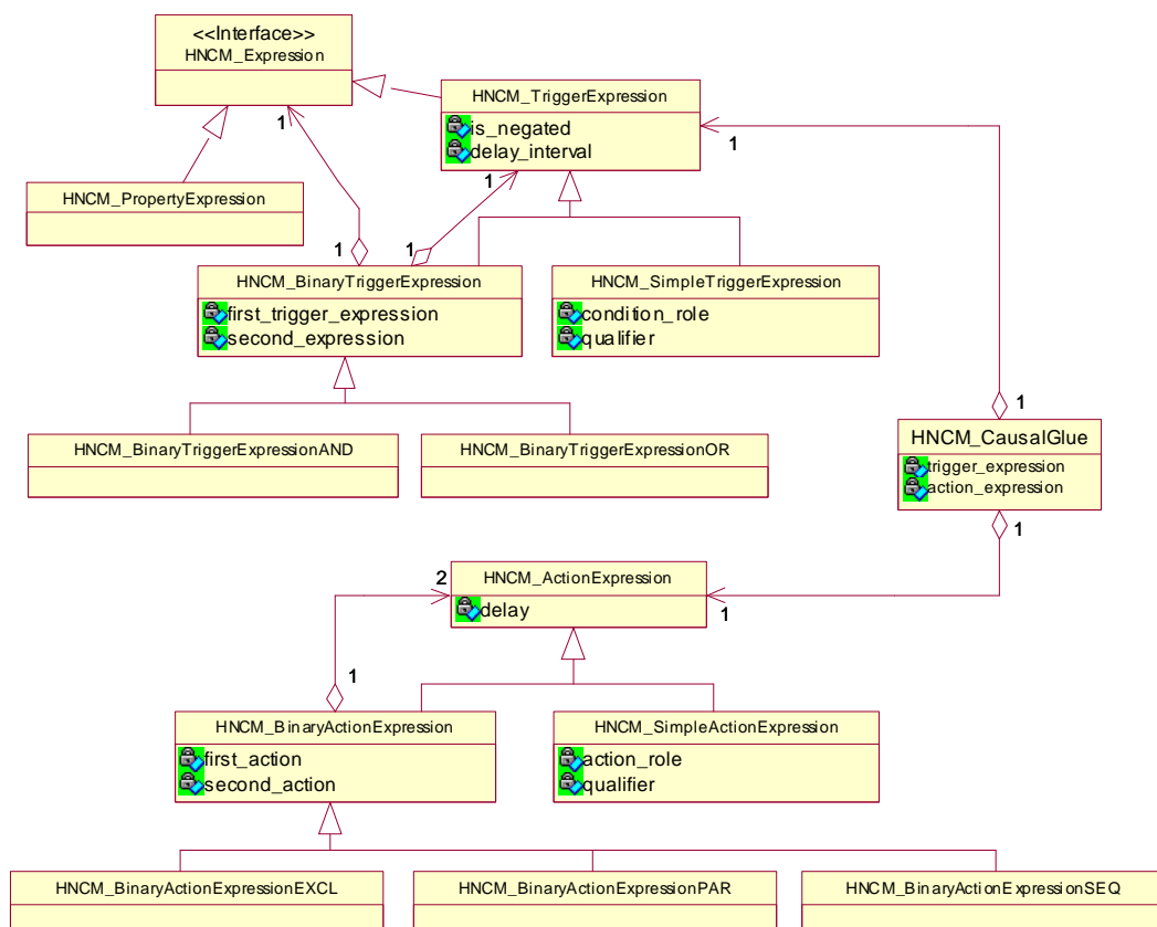
Figura 37. Diagrama de classes para glue do tipo causal
