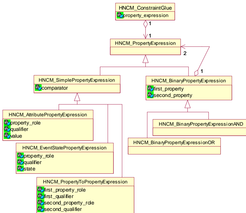
Figura 36. Diagrama de classes para glue do tipo restrição
