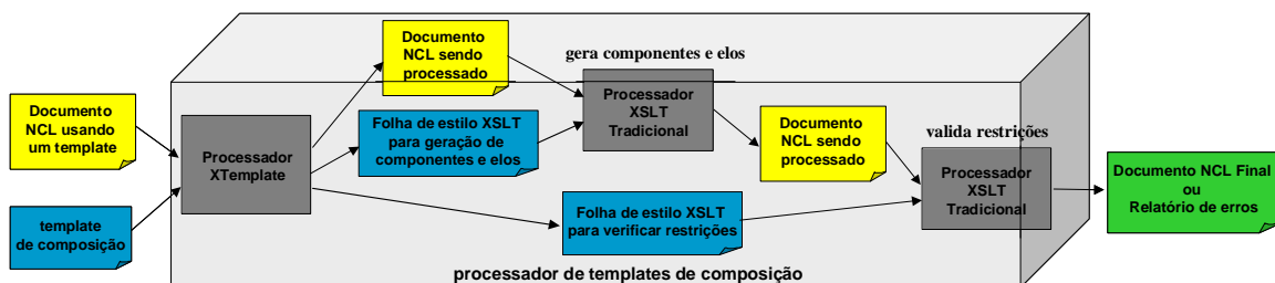
Figura 48. Estrutura detalhada do futuro processador de templates de composição
