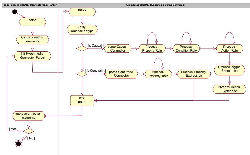
Figura 41. Diagrama de atividades do HXML_ConnectorBaseParser
