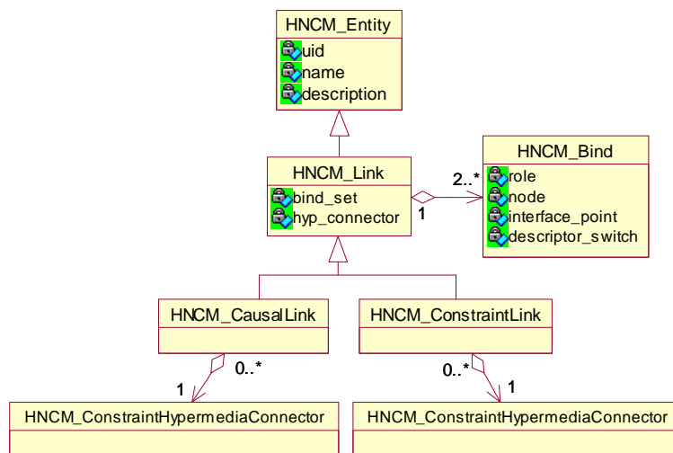
Figura 38. Diagrama de classes para entidade elo
