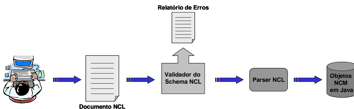
Figura 39. Processo declarativo de autoria no sistema HyperProp
