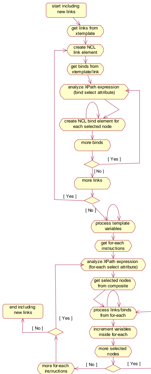
Figura 46. Diagrama de atividades do método includeLinks
