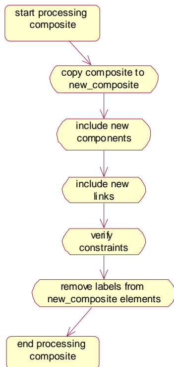
Figura 45. Diagrama de atividades do método processComposite
