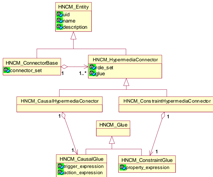
Figura 34. Diagrama de classes para entidade conector hipermídia
