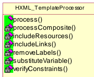
Figura 43. Classe HXML_TemplateProcessor
