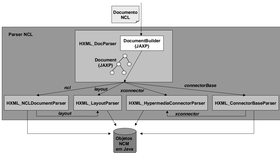
Figura 40. Estrutura do Parser NCL
