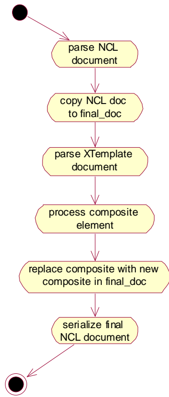
Figura 44. Diagrama de atividades do método process
