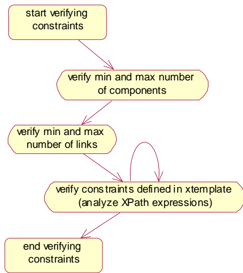
Figura 47. Diagrama de atividades do método verifyConstraints
