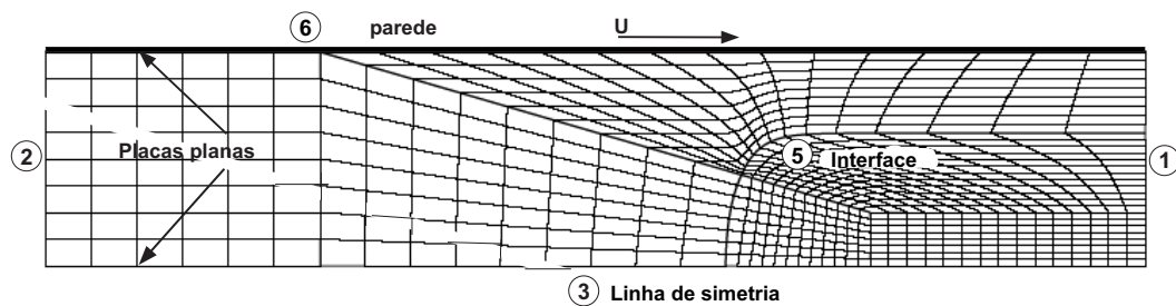
Figura 5.4: Diagrama esquemático com as condições de contorno do problema do escoamento de uma gota infinita num capilar reto.
