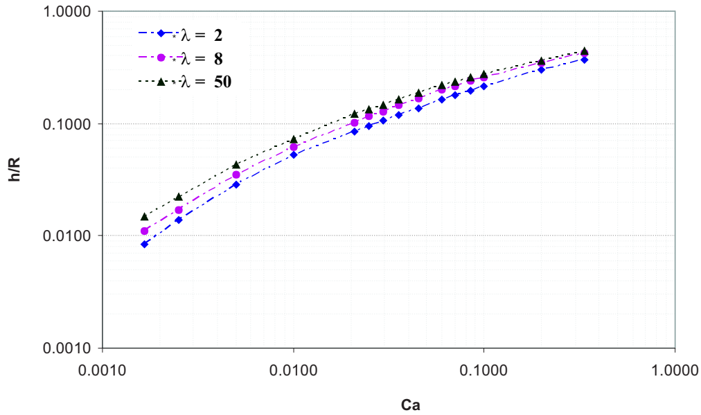
Figura 5.9: Espessura da capa de líquido remanescente em função do número de capilaridade.
