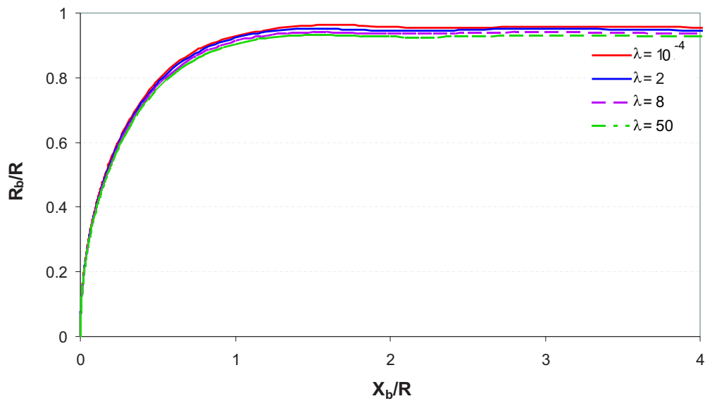
Figura 5.10: Perfis da interface para Ca = 0.01 e distintas razões de viscosidade \lambda .
