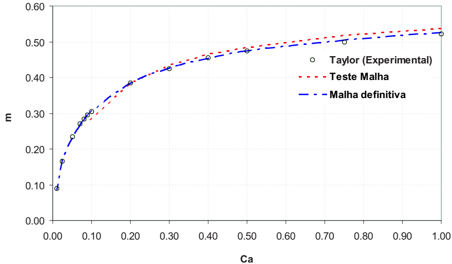
Figura 5.7: Comparação dos valores de m calculados usando as malhas testadas e valores experimentais de Taylor.
