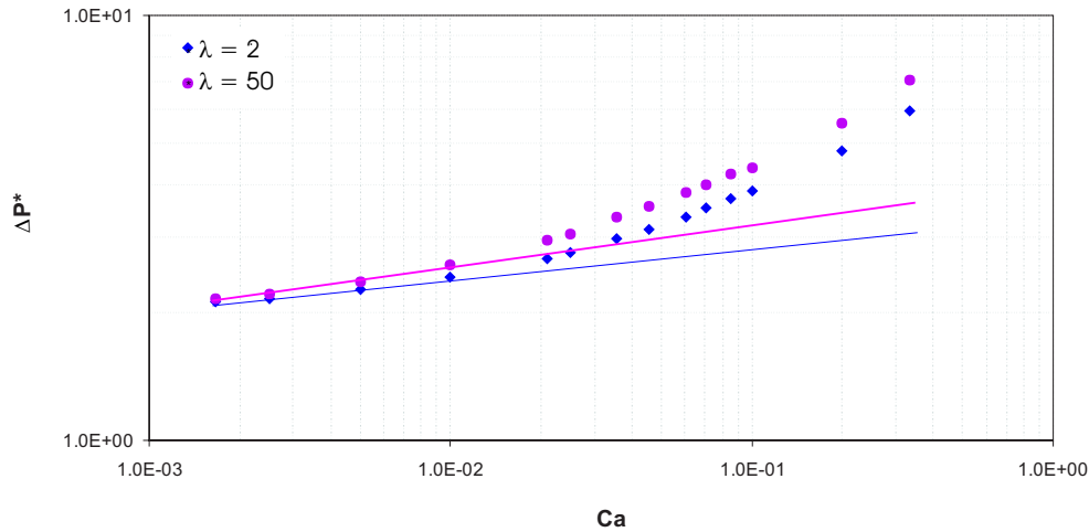
Figura 5.15: Queda de pressão adimensional em função do número Ca para \lambda = 2 e 50 . Linhas assintóticas com valores de m de 42.4 e 60.3 respectivamente.
