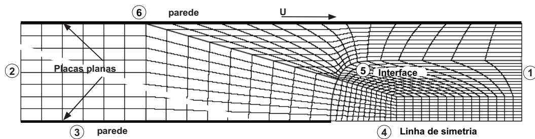
Figura 5.3: Segundo passo para a solução do problema do escoamento de uma gota num capilar reto.
