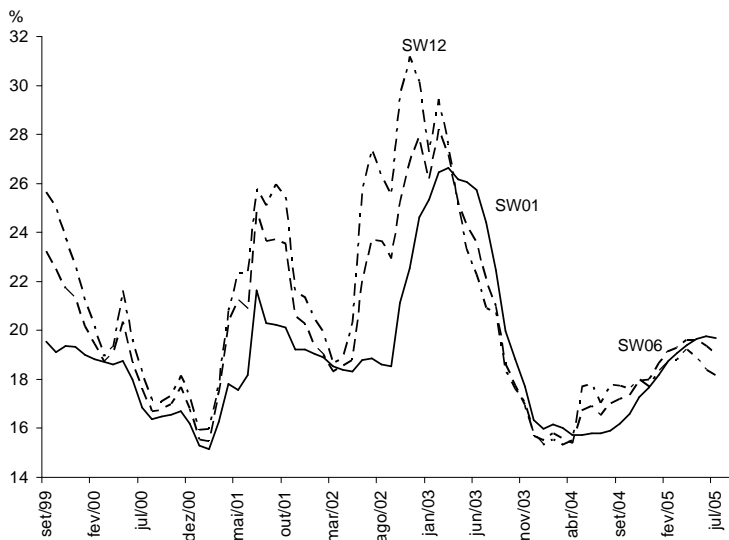
Figura 1.3: Evolução das taxas para diferentes maturidades
